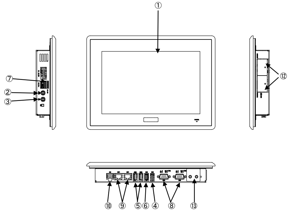
図 3-1-2. 外形図 (APS4-101BN)
