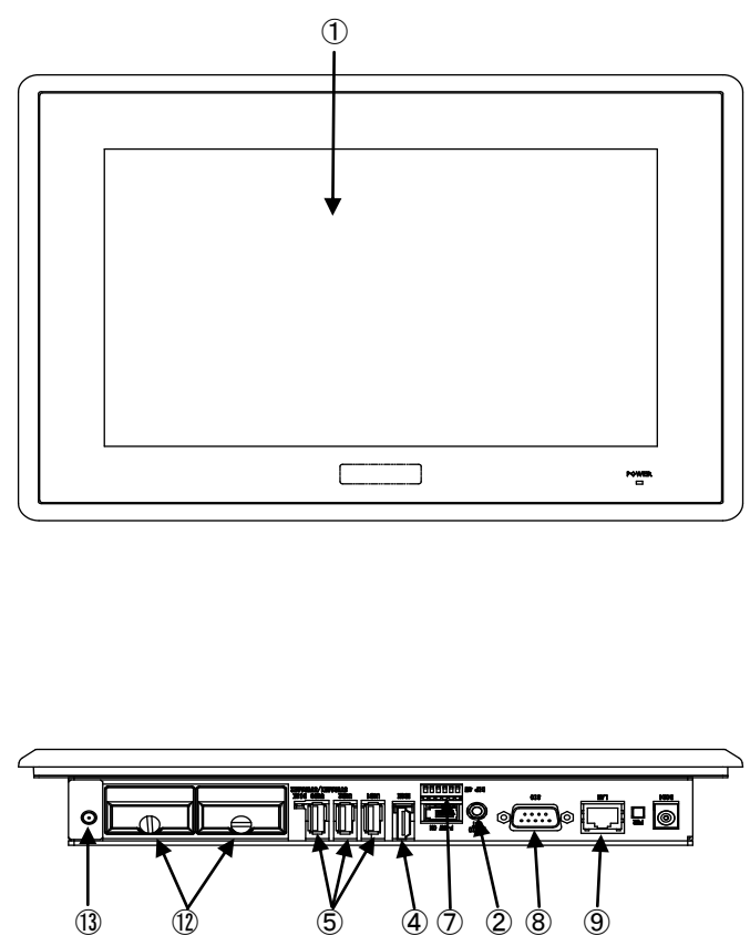
図 3-1-3. 外形図 (APL4-101BN)
