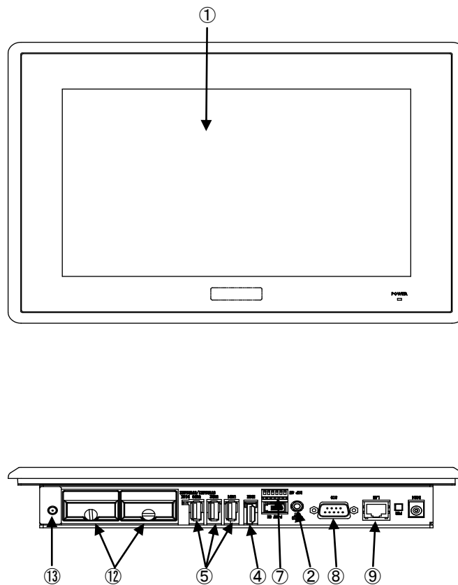
図 3-1-3. 外形図 (APL4-101BN)
