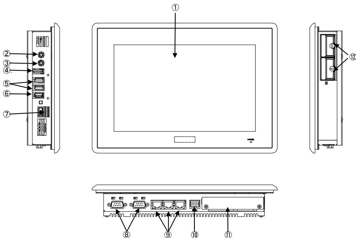
図 3-1-1. 外形図 (AP4-101AN)
