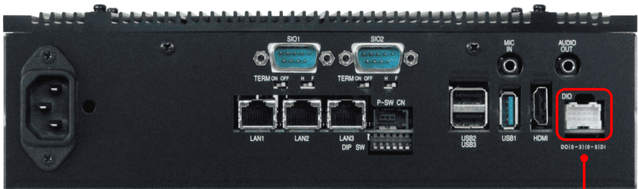
DIO インタフェースコネクタ(DIO)
