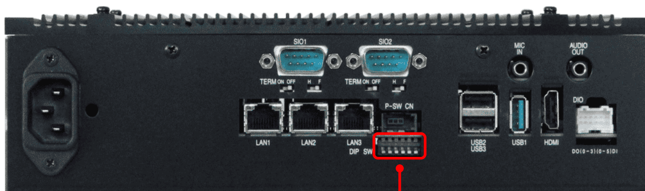
MODE 設定スイッチ (DIP SW)
