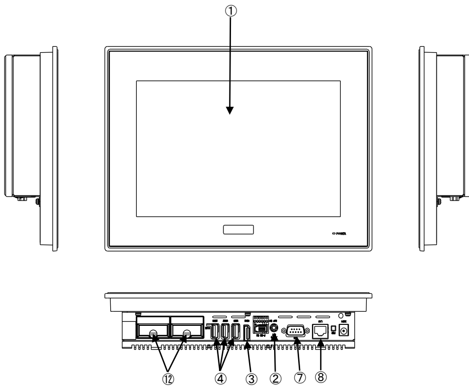
図 4-3. 外形図 (APL4A-101BN)
