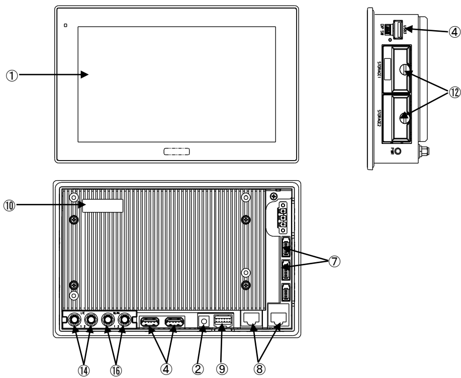
図 4-7. 外形図 (APS4A-070DN/DS)
