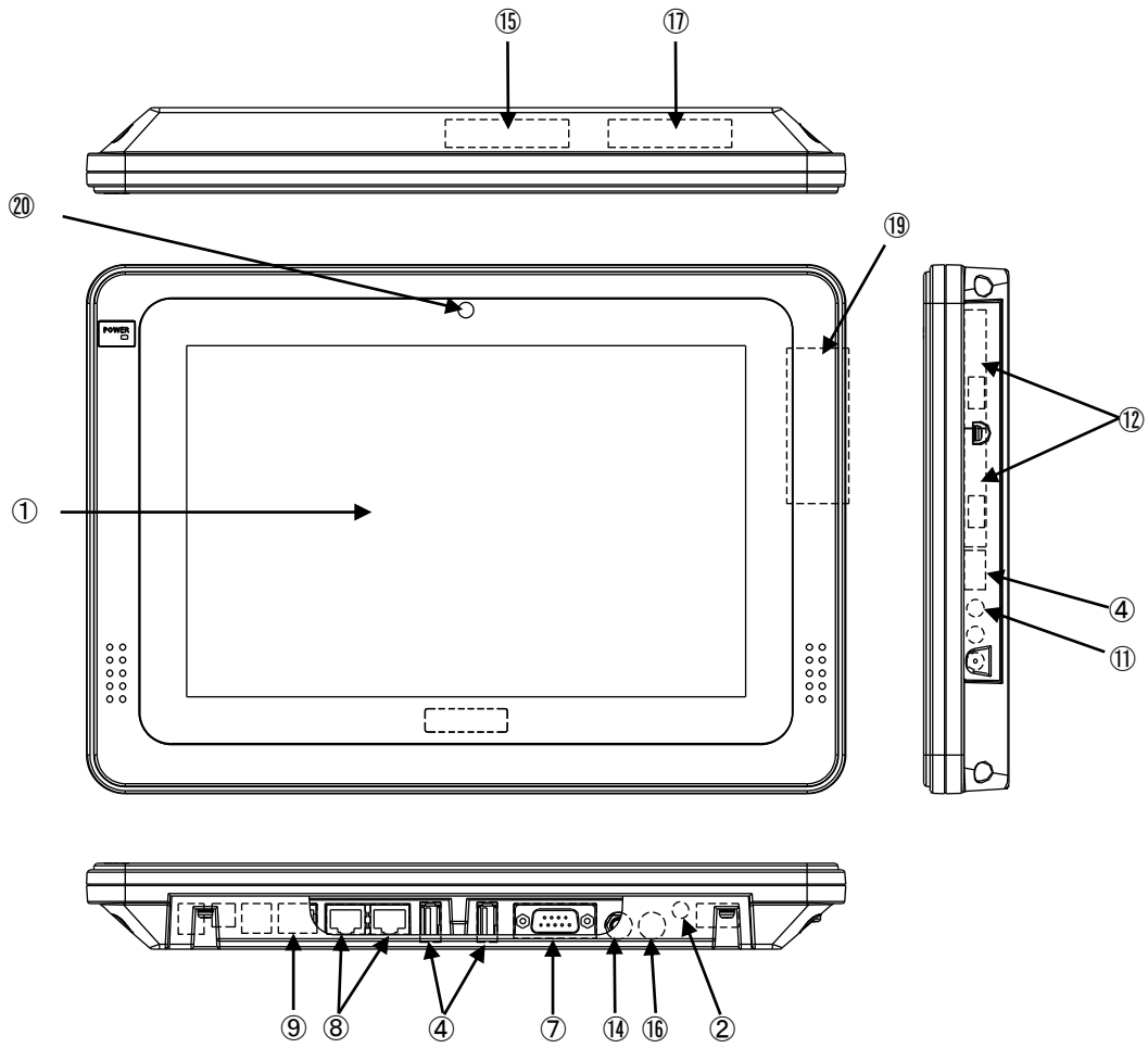
図 4-8. 外形図 (AS4A-101DN/DS)
