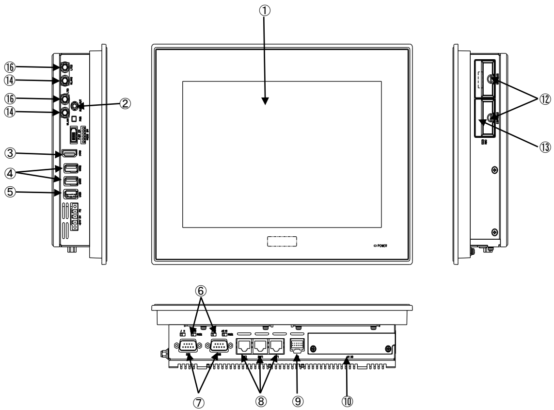
図 4-5. 外形図 (AP4A-101CN)
