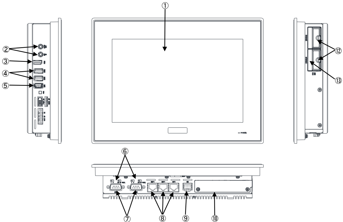
図 4-1. 外形図 (AP4A-101AN)
