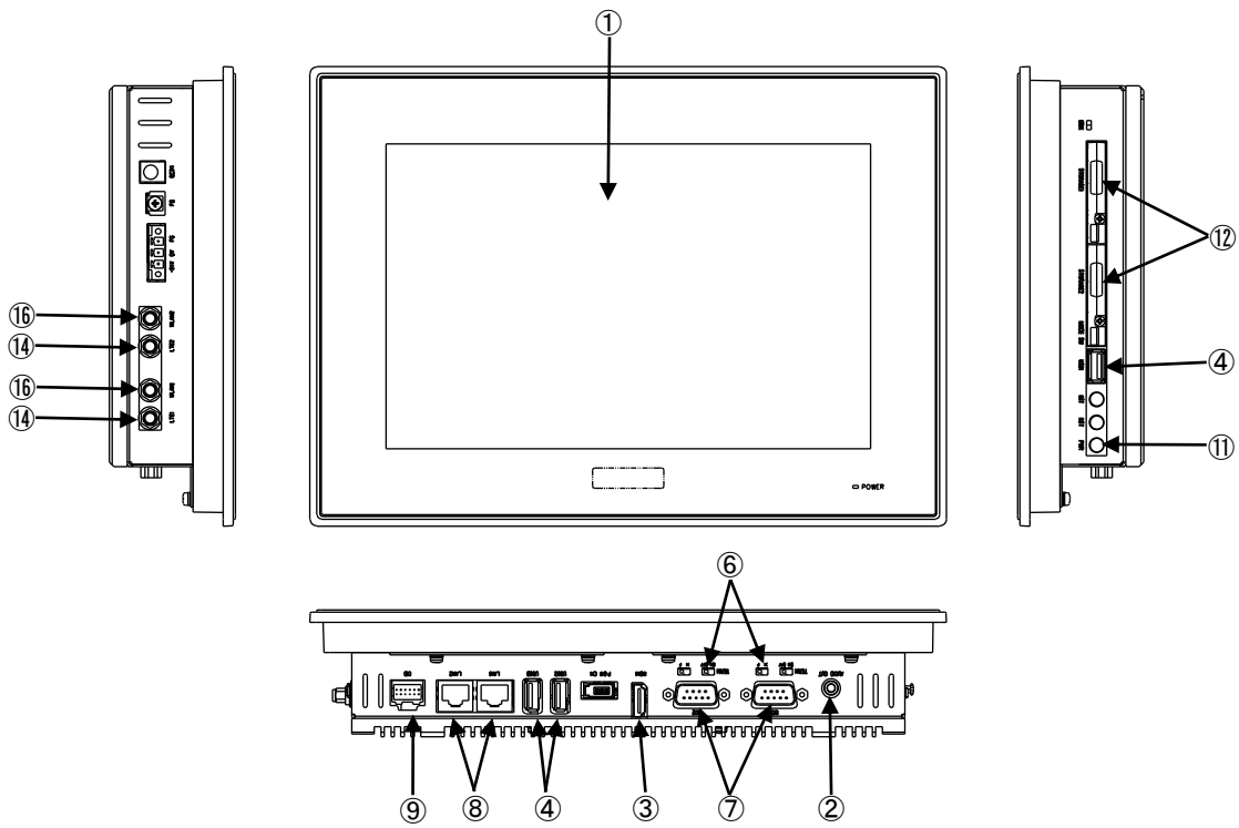
図 4-6. 外形図 (APS4A-101DN)
