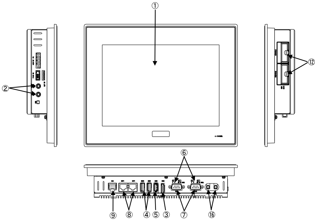
図 4-2. 外形図 (APS4A-101BN)
