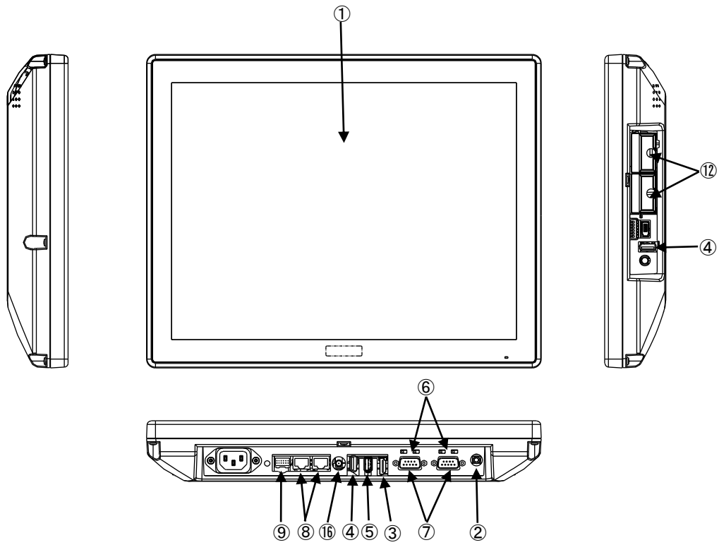
図 4-4. 外形図 (AS4A-150BNA)
