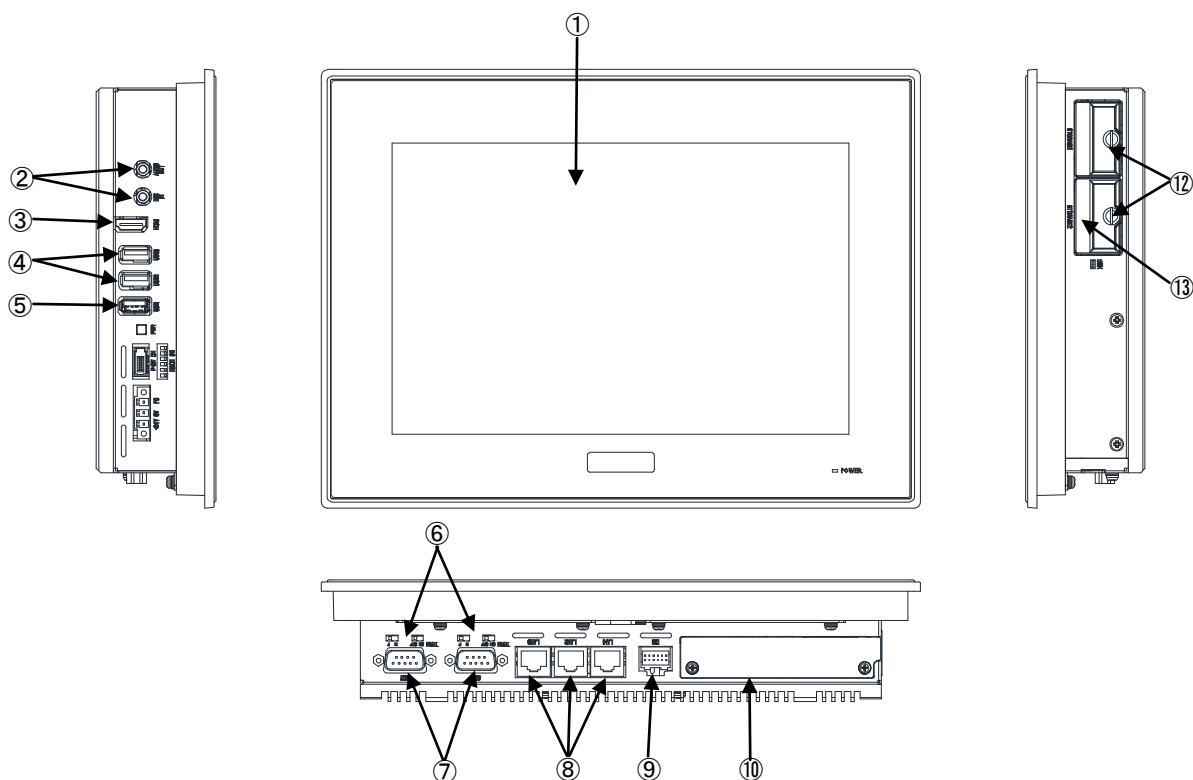
図 3-1-1. 外形図 (AP4A-101AN)
