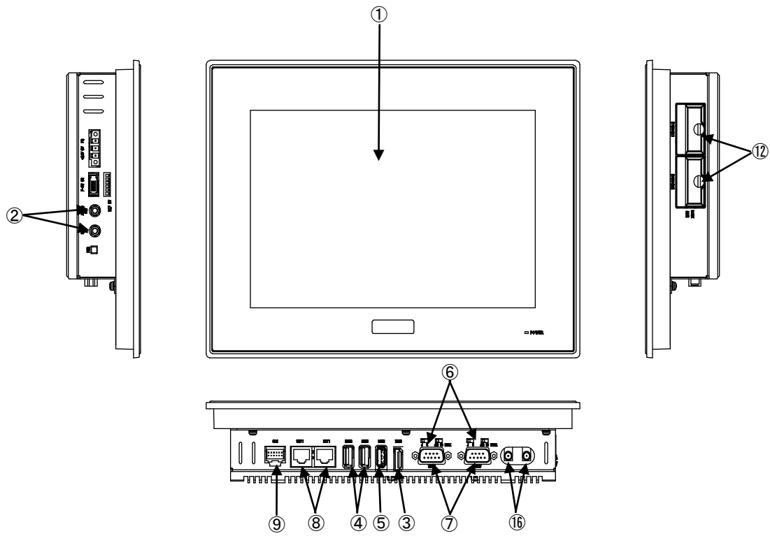
図 3-1-2. 外形図 (APS4A-101BN)
