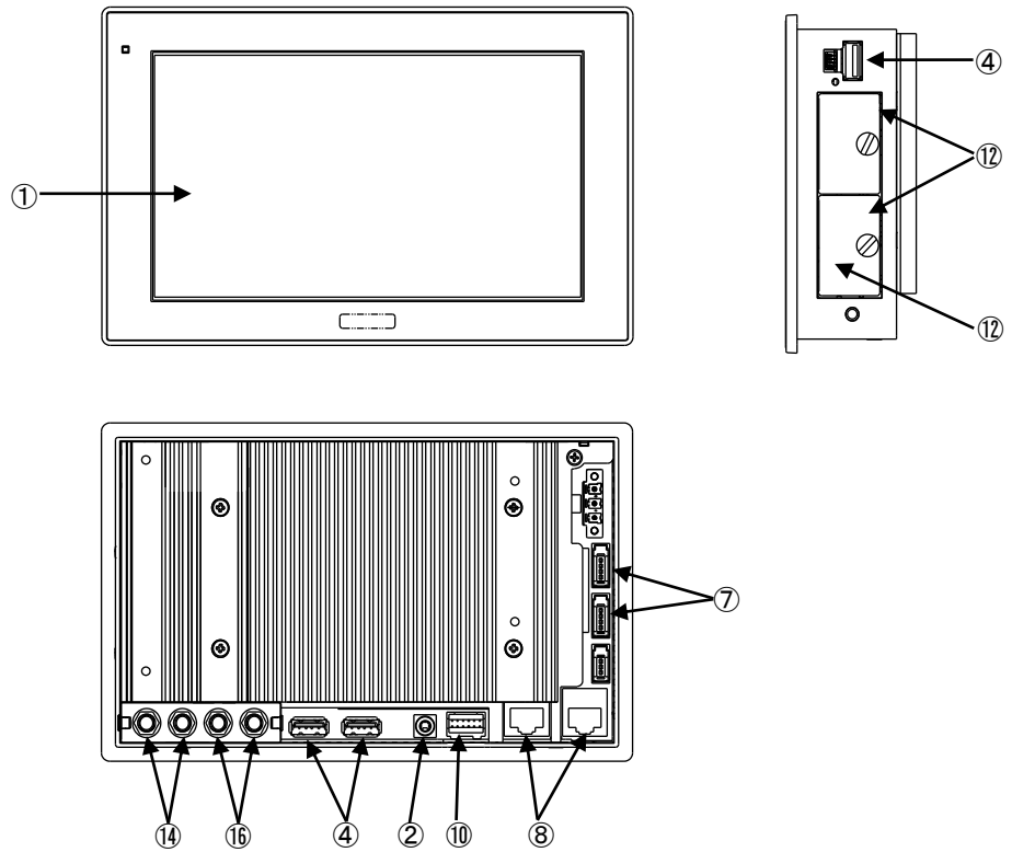
図 4-3. 外形図 (APS4A-070DN/DS)
