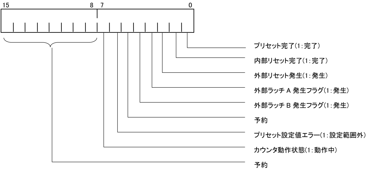
図 4-1-2-1 ステータス割付
