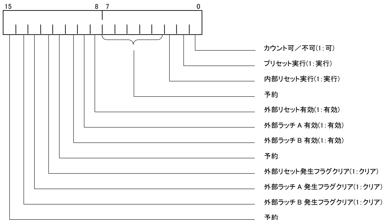
図 4-1-2-2 ソフトスイッチ割付
