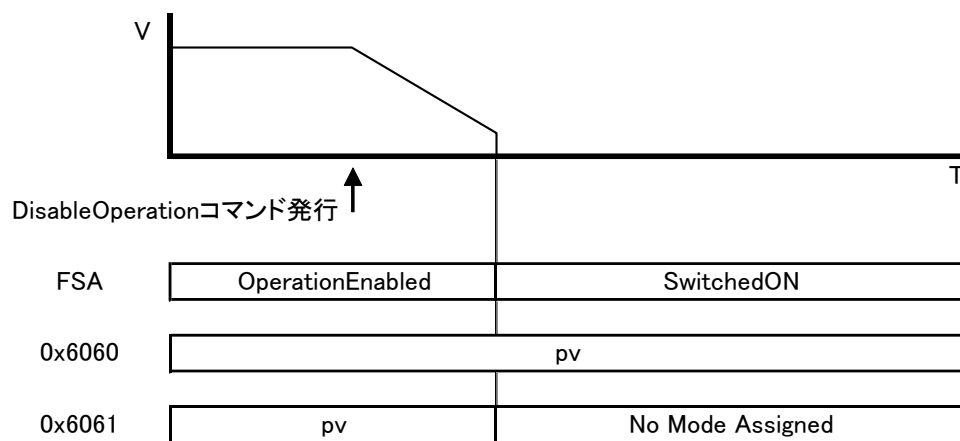
図 4-3-4-1 プロファイル速度モード実行中に DisableOperation コマンド実行したときの例
