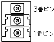
DC24V 電源供給コネクタ (PWR1, PWR2)
