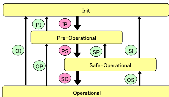
図 3-5-4-1 EtherCAT State Machine
