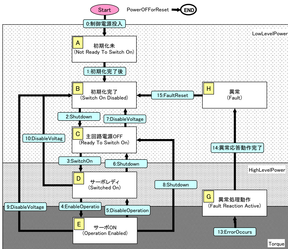
図 4-3-1-1 EtherCAT CiA402 状態遷移図
