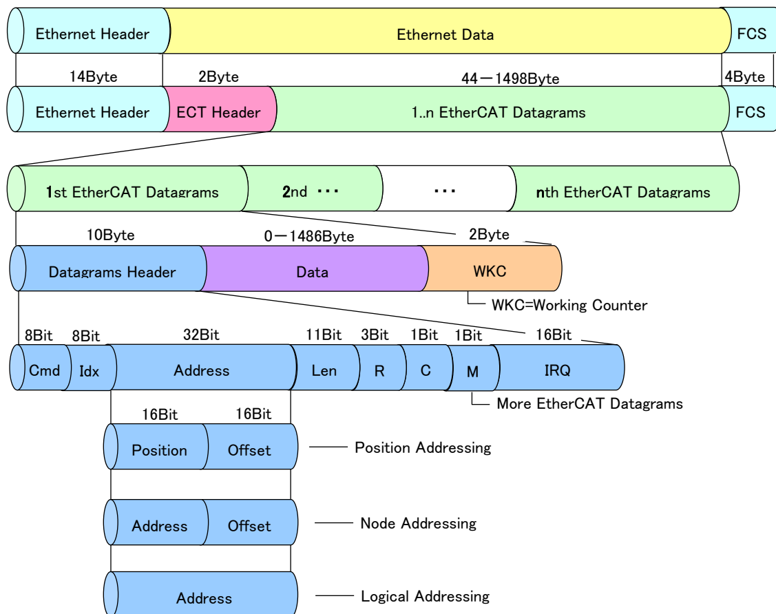
図 3-5-2-2 EtherCAT Datagram
