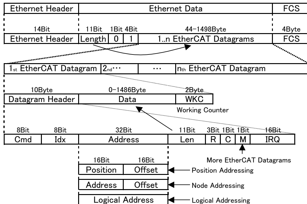
図 3-3-2-2 EtherCAT Datagram
