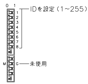
ディップスイッチ
