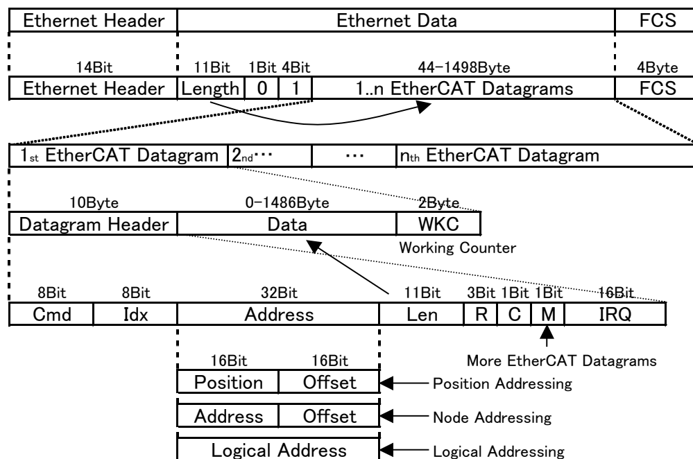
図 3-3-2-2 EtherCAT Datagram
