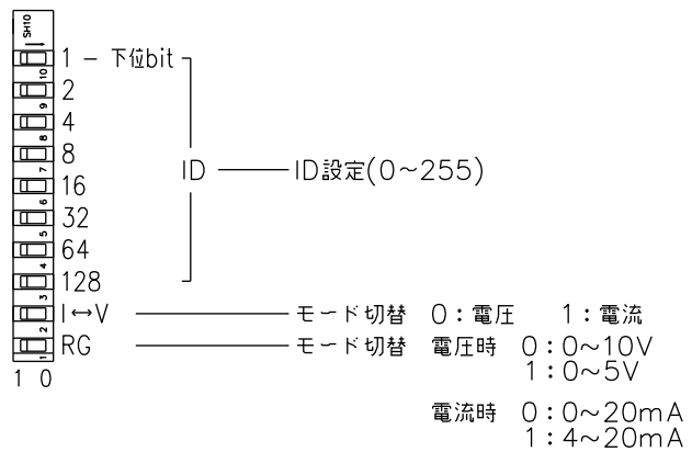
ディップスイッチ
