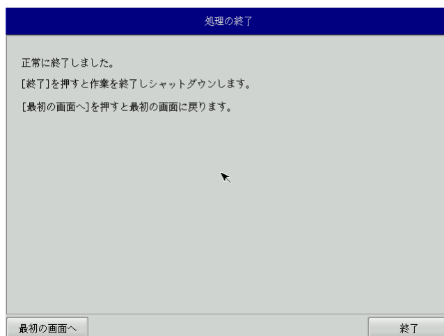
図 6-4-7. 終了画面
