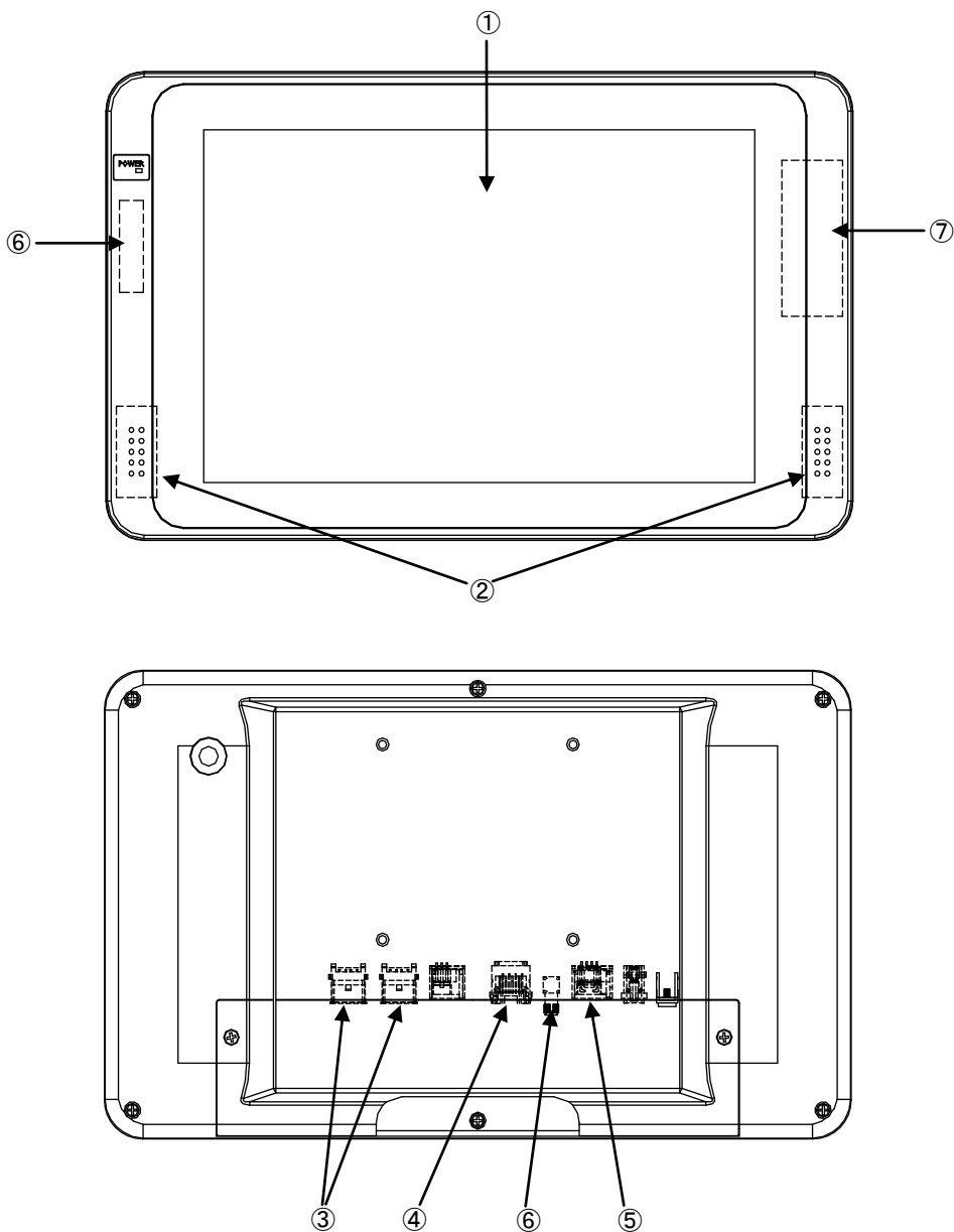
図 3-1-1. 外形図 (MT4-101BNA)
