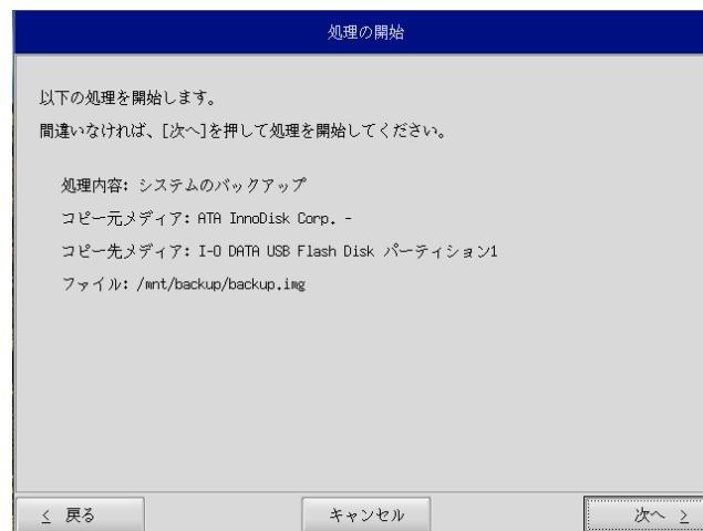
図 6-4-5. 確認画面
