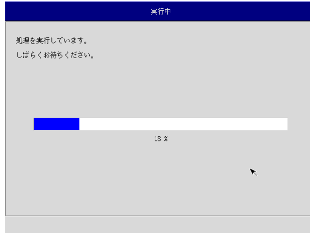
図 6-2-6. 実行中画面
