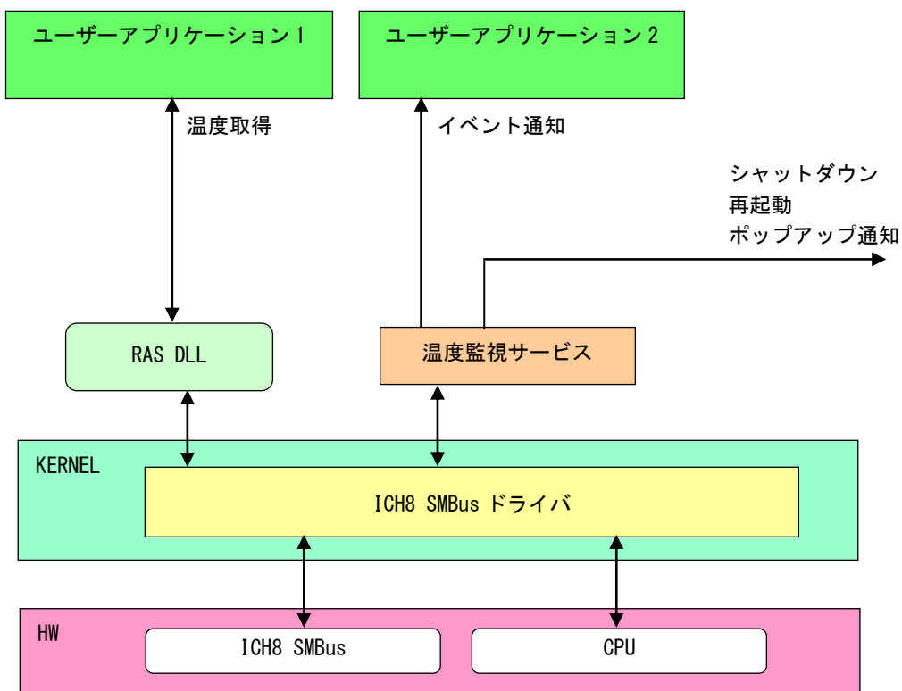
図 5-6-2-1. RAS DLL
