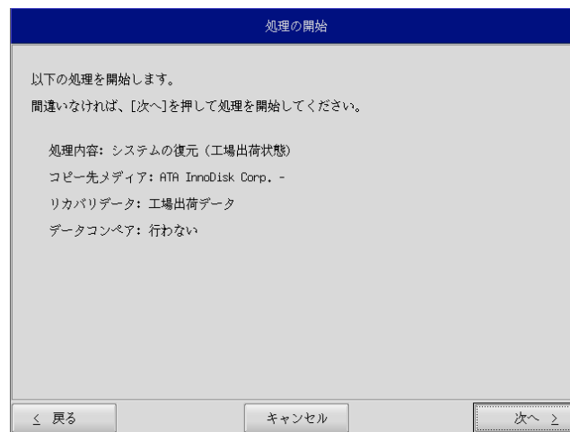
図 6-2-5. 確認画面
