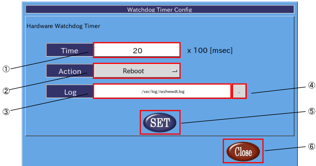
図 2-3-7-1. ハードウェア・ウォッチドッグタイマの設定
