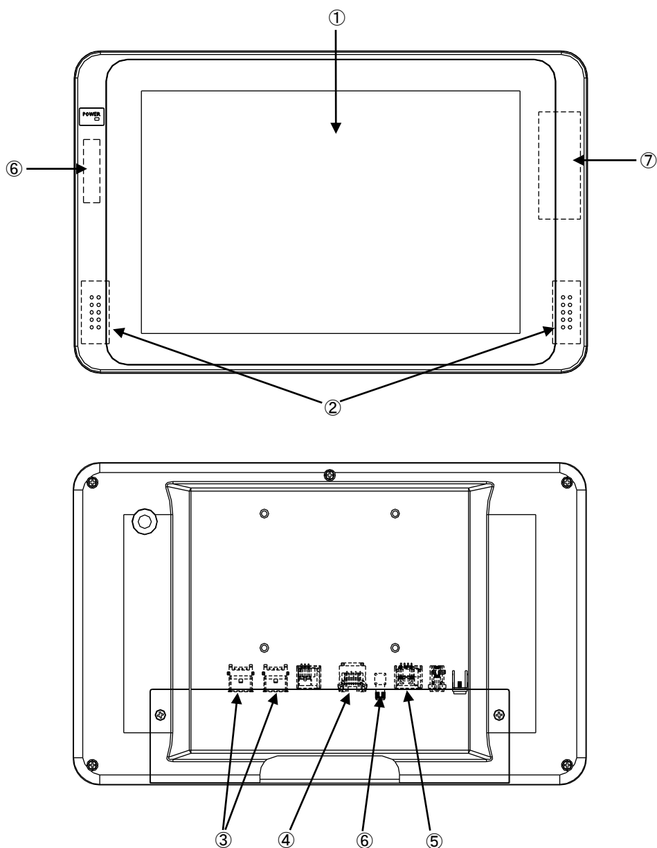
図 4-1. 外形図 (MT4-101BN)
