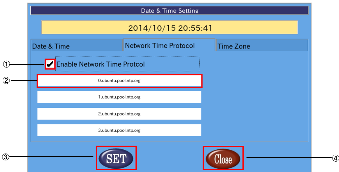
図 2-3-5-2. NTP サーバの設定
