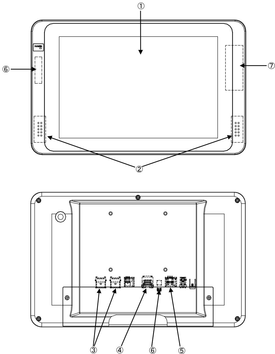
図 4-1. 外形図 (MT4-101CN)
