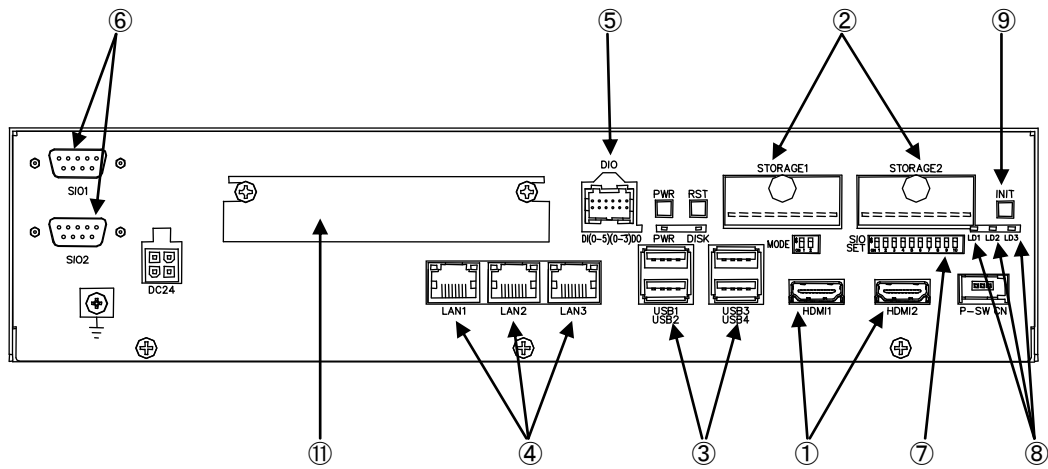
図 3-1-2. 外形図 (FC4-100A)
