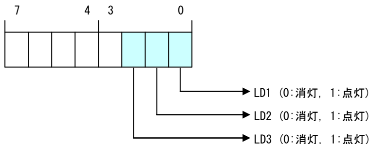
図 5-7-1-2. 汎用 LED データ
