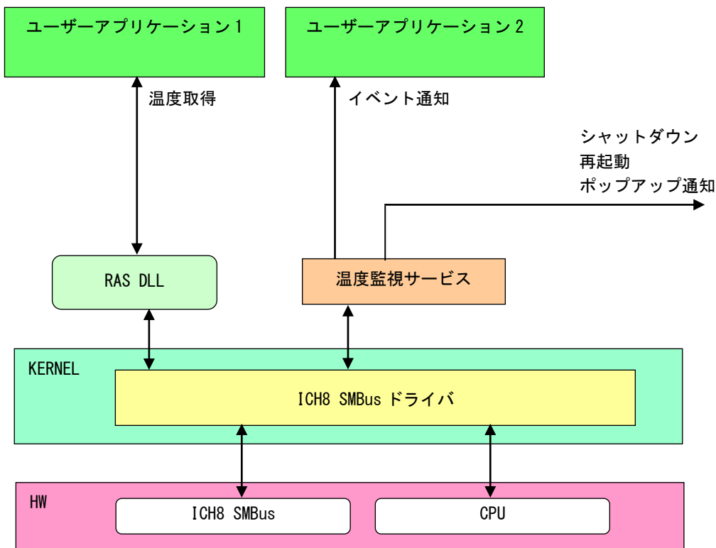
図 5-10-2-1. RAS DLL
