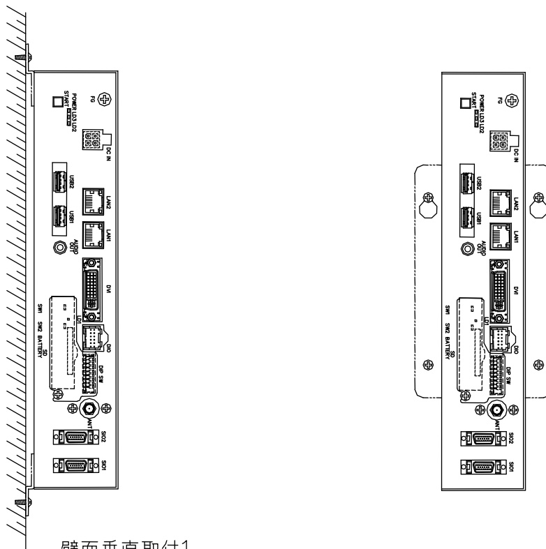
壁面垂直取付1
