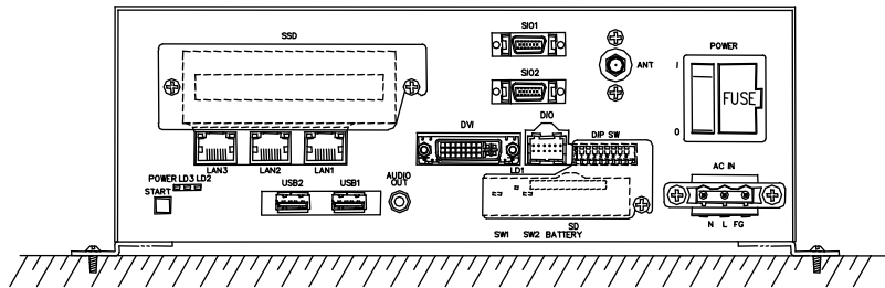
床面水平取付
