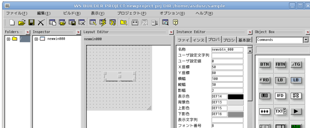
図 3-3-4-2. アプリケーションウィンドウに配置されたボタン
