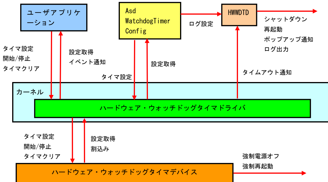
図 4-3-4-1. ハードウェア・ウォッチドッグタイマの構成
