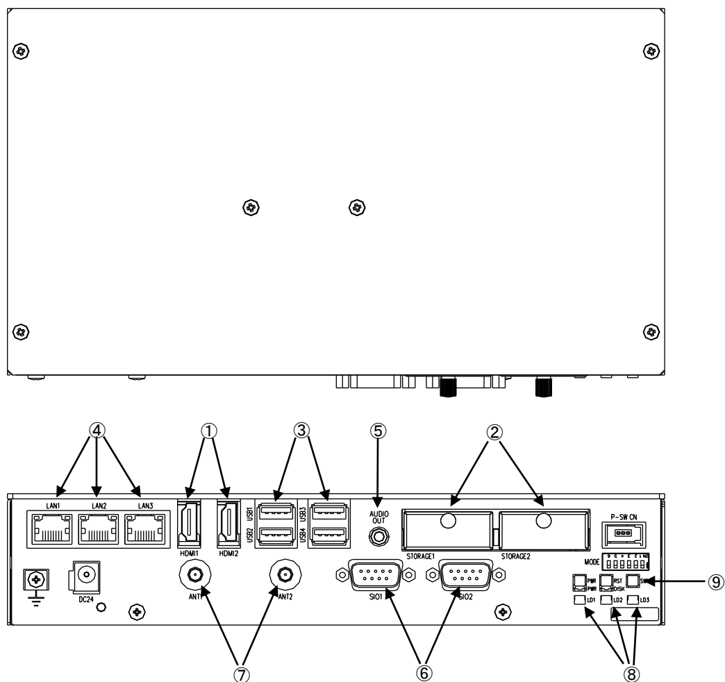
図 4-1. 外形図 (ECL4-100B-**-W)
