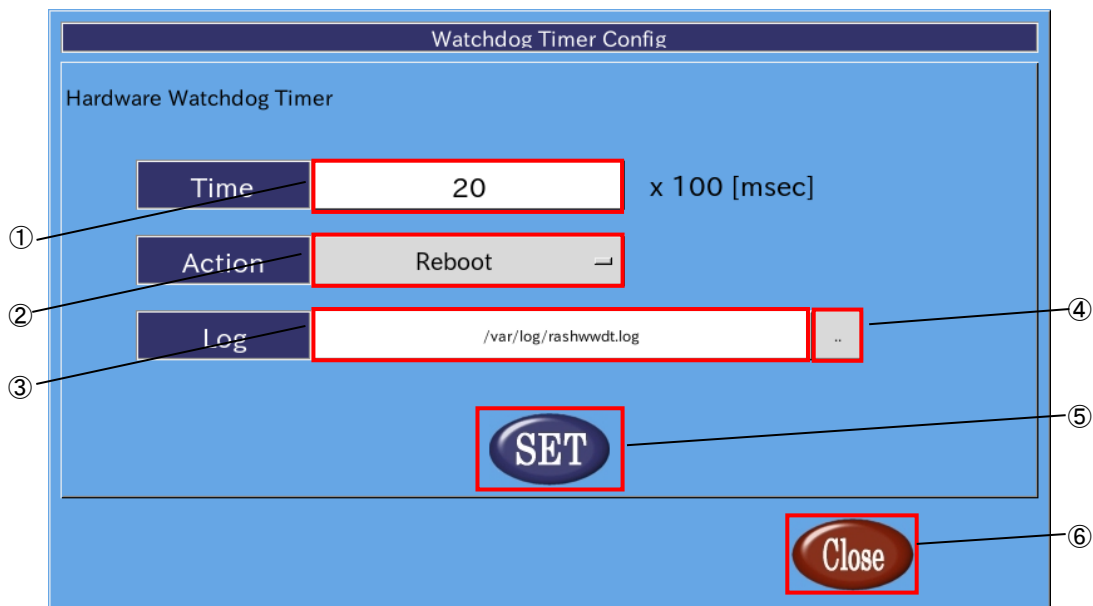
図 2-3-7-1. ハードウェア・ウォッチドッグタイマの設定
