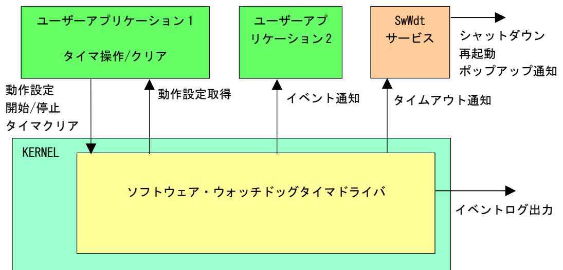
図 5-6-2-1. ソフトウェア・ウォッチドッグタイマドライバ
