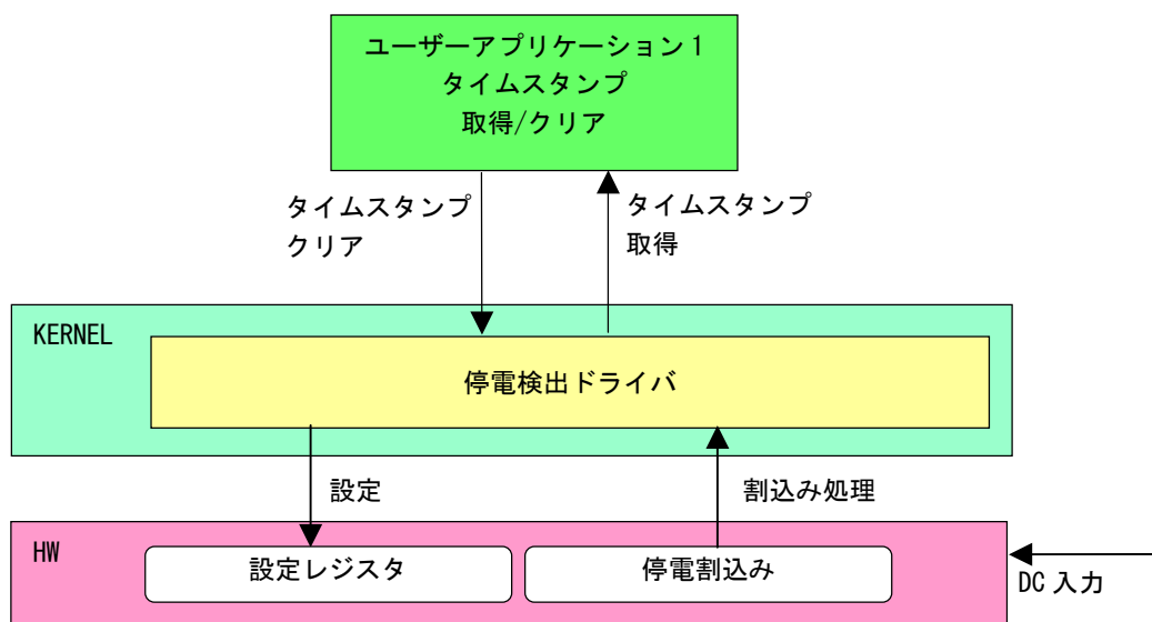
図 5-9-2-1. 停電検出ドライバ
