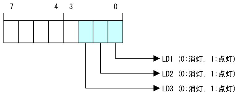
図 5-4-1-2. 汎用 LED データ
