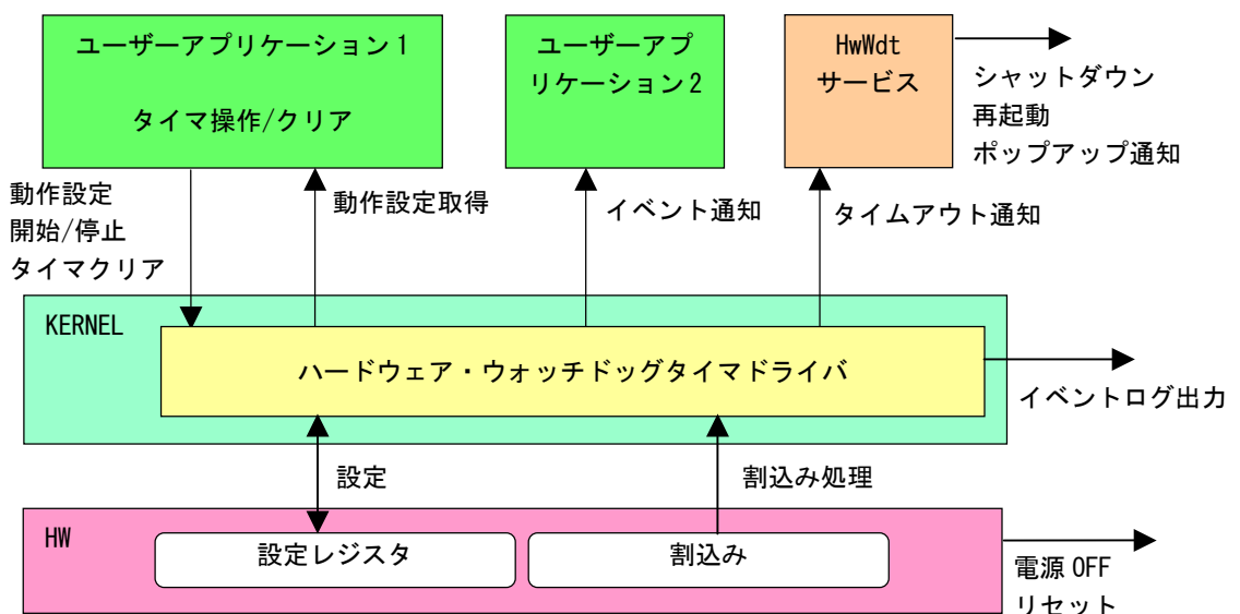
図 5-5-2-1. ハードウェア・ウォッチドッグタイマドライバ
