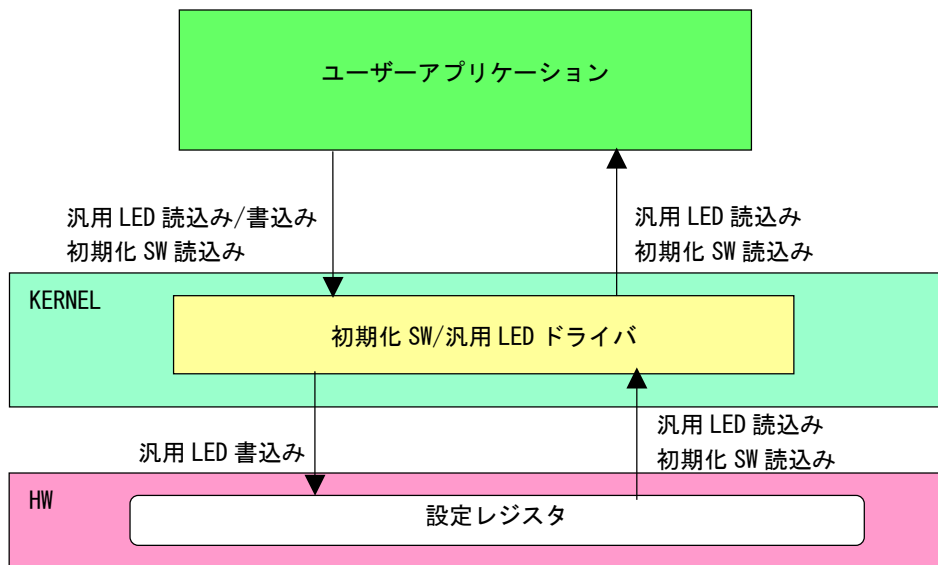
図 5-4-2-1. 初期化 SW/汎用 LED ドライバ
