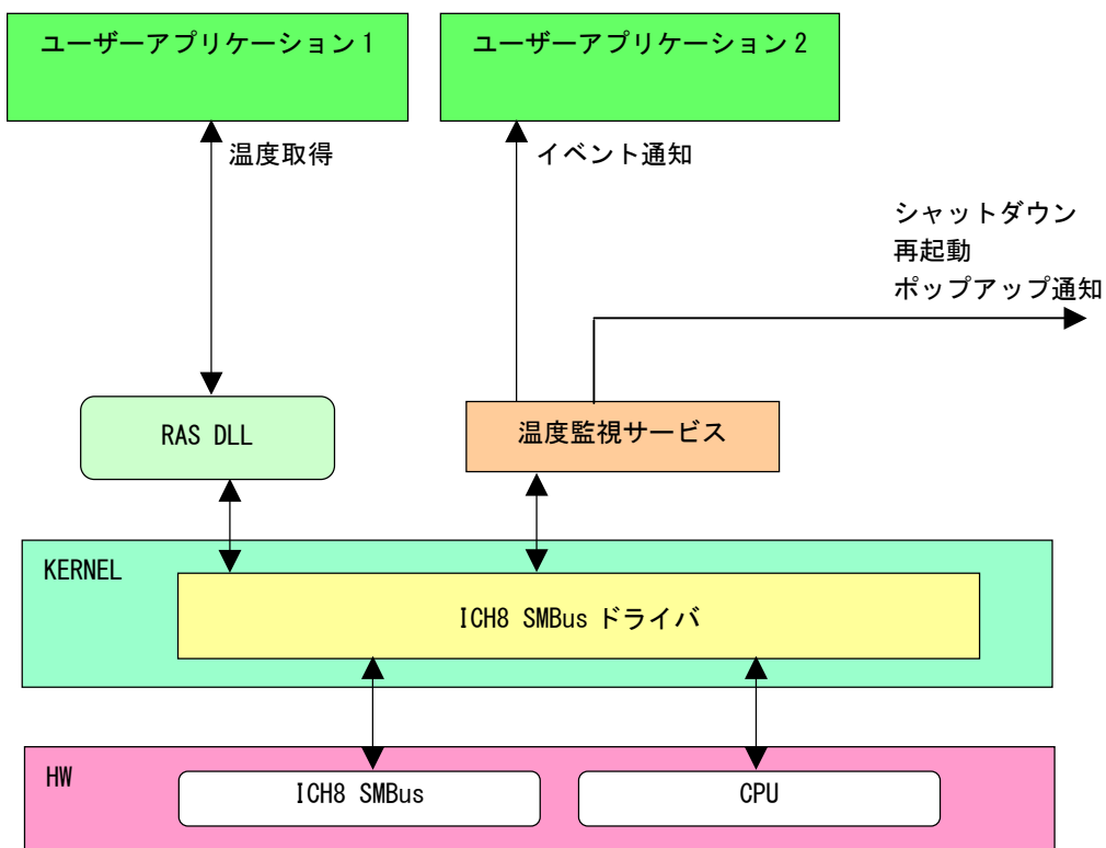
図 5-7-2-1. RAS DLL
