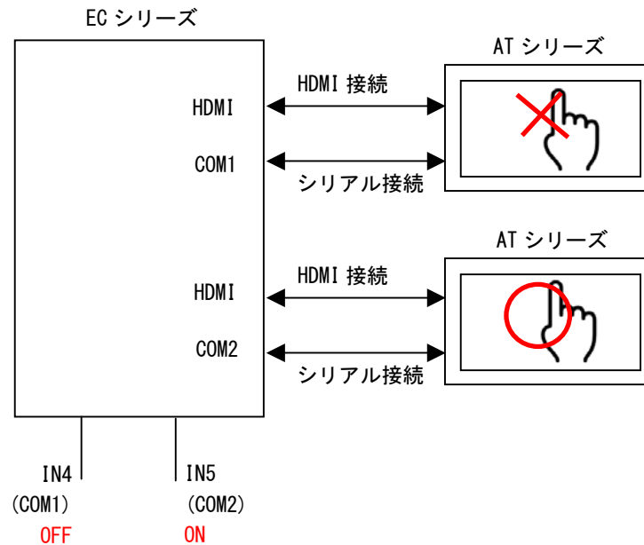
図 2-7-5-2. タッチパネルインターロック IN4→OFF、IN5→ON
