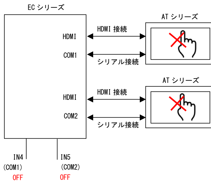
図 2-7-5-4. タッチパネルインターロック IN4→OFF、IN5→ON
