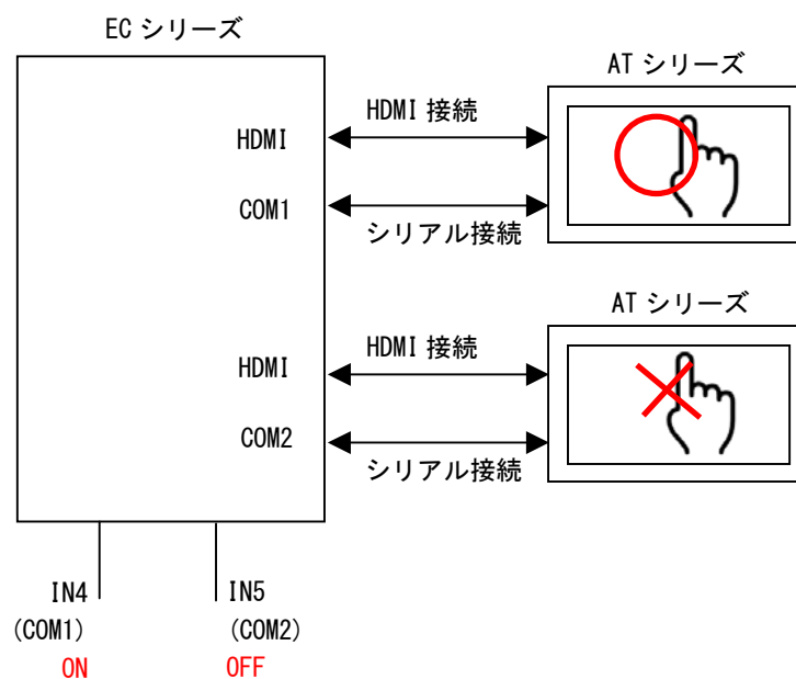
図 2-7-5-3. タッチパネルインターロック IN4→ON、IN5→OFF
