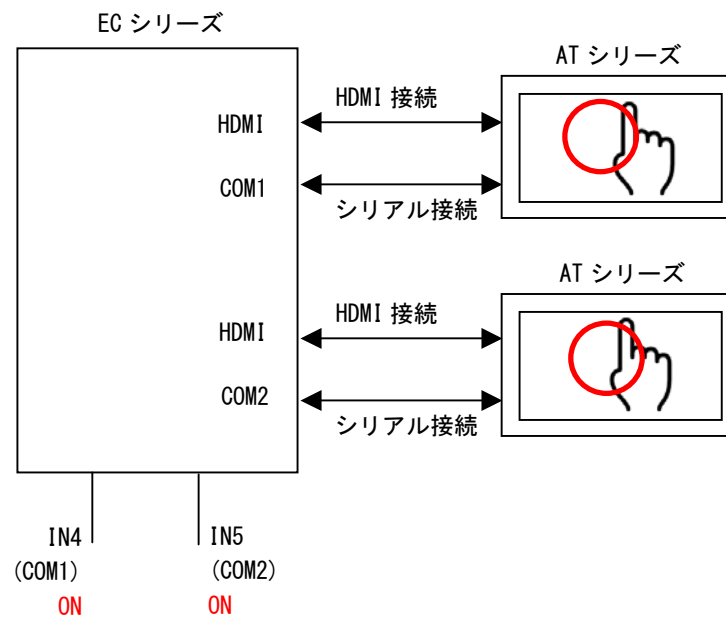
図 2-7-5-1. タッチパネルインターロック IN4→ON、IN5→ON
