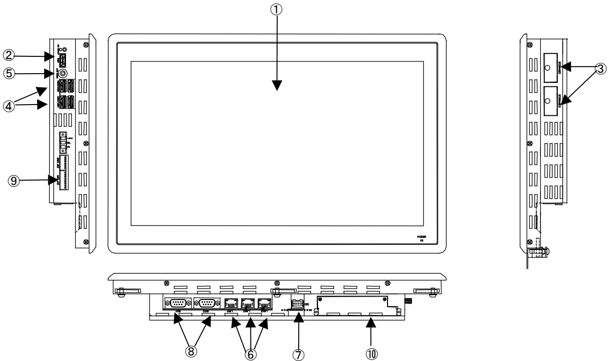
図 3-1-5. 外形図 (AP7-156B*/AP7-156C*)
