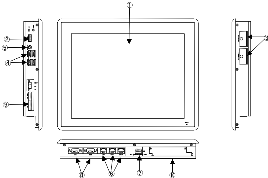
図 3-1-1. 外形図 (AP7-121B*/AP7-121C*)
