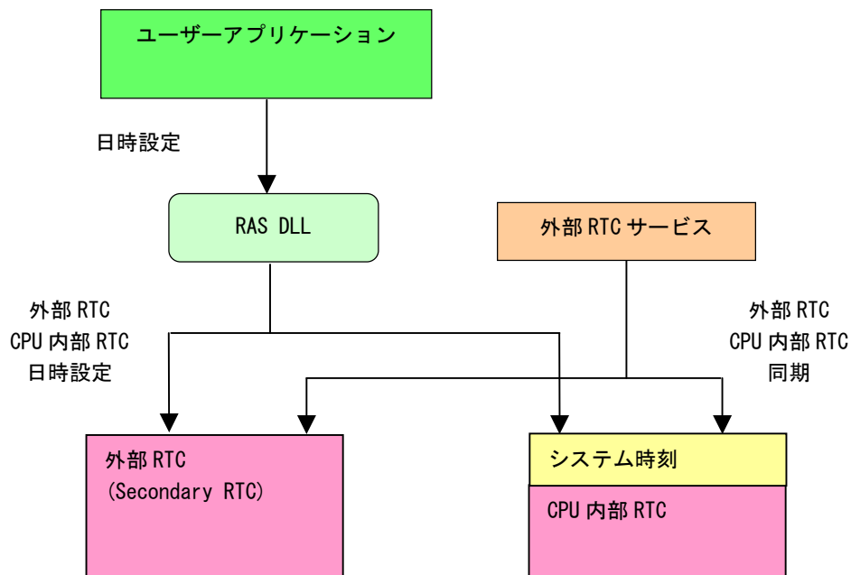
図 5-12-2-1. RAS DLL 日時設定
