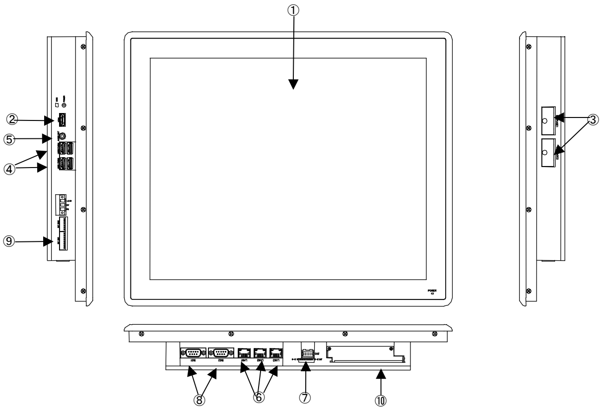
図 3-1-3. 外形図 (AP7-170B*/AP7-170C*)
