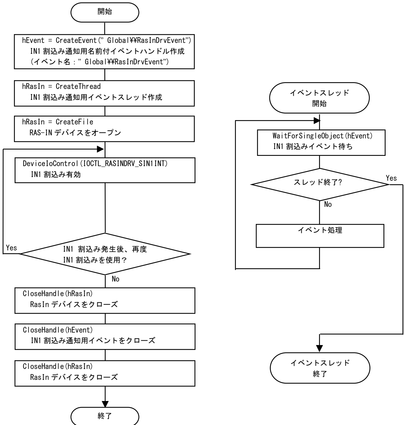
図 5-6-4-1. IN1 割込み仕様手順
