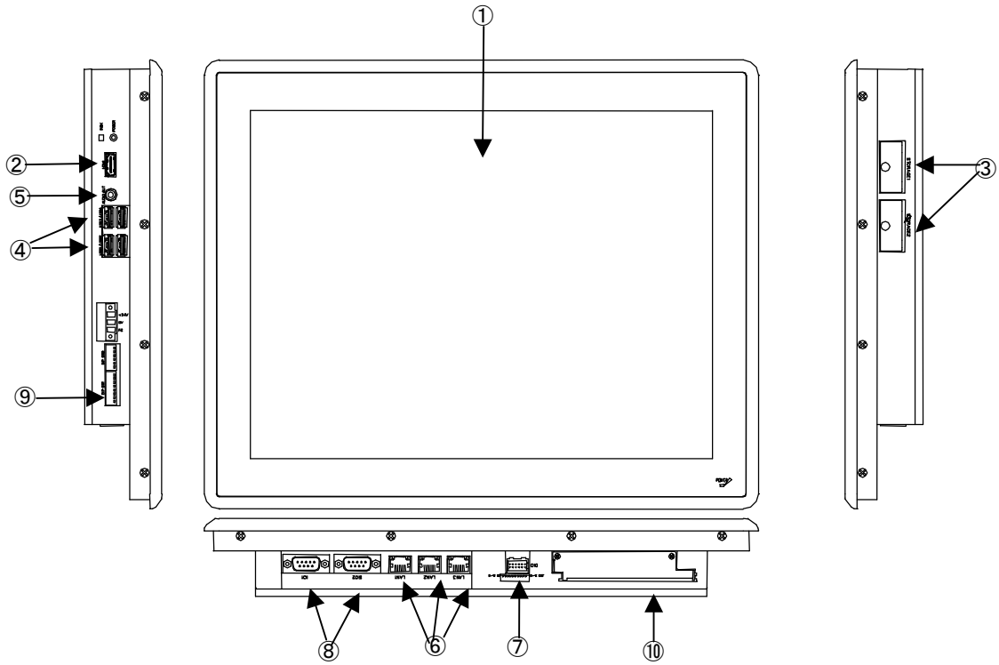
図 3-1-2. 外形図 (AP7-150B*/AP7-150C*)
