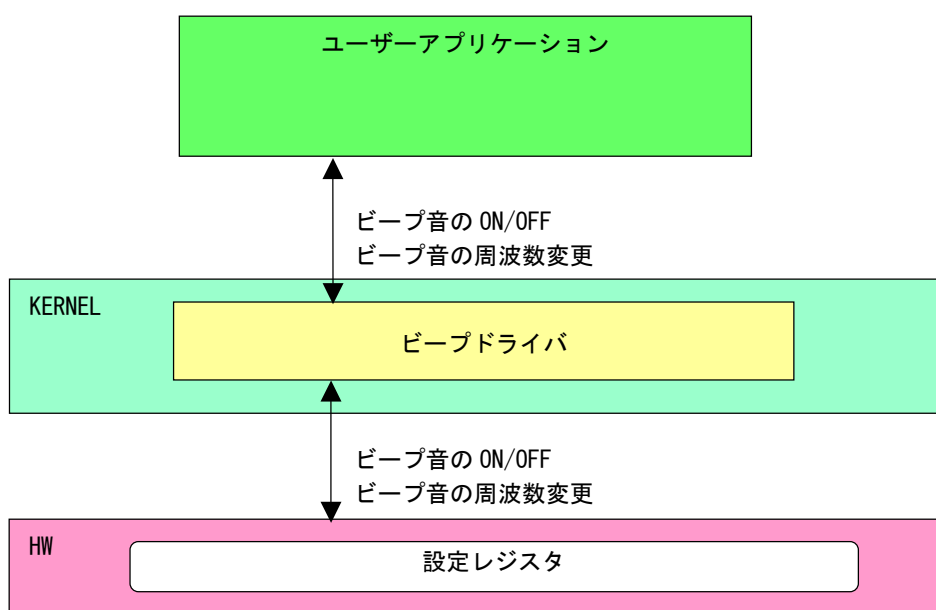
図 5-14-2-1. ビープドライバ
