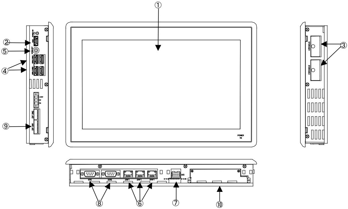
図 3-1-4. 外形図 (AP7-116B*/AP7-116C*)
