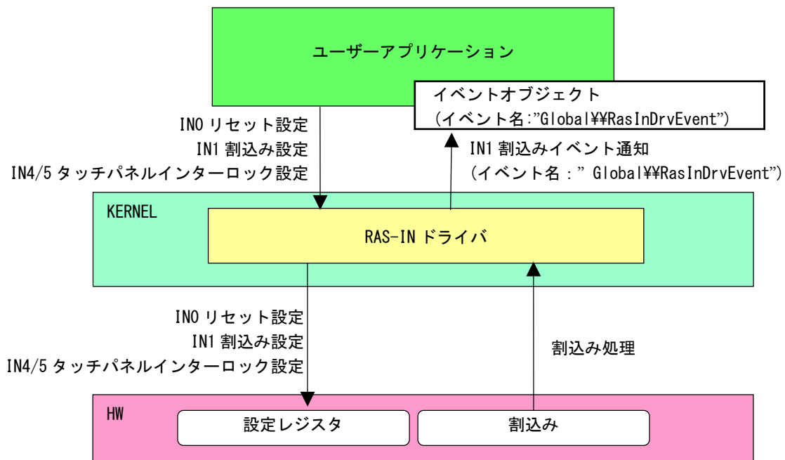
図 5-6-2-1. RAS-IN ドライバ
