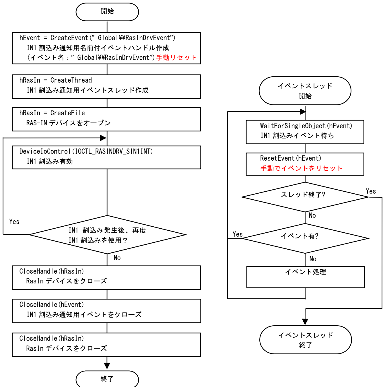
図 5-6-5-1. 複数アプリケーションで IN1 割り込みを使用する手順
