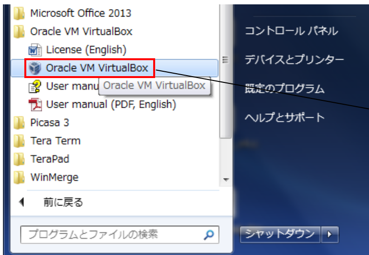
図 3-2-4-1. VirtualBox 起動
