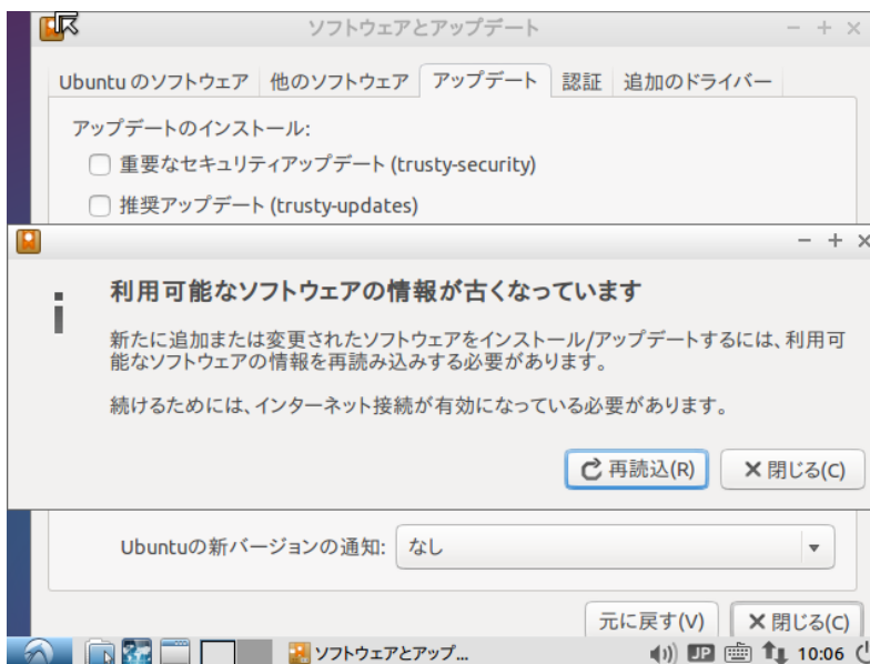
図 3-5-4-3. 確認画面
