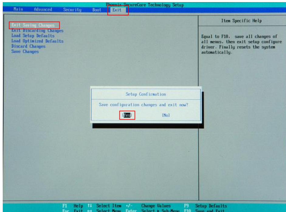
図 5-2-1-6. BIOS 設定 保存と終了
