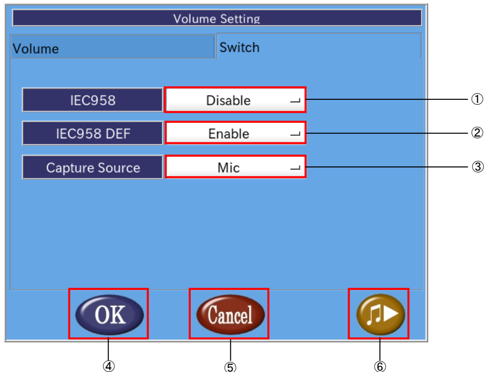
図 2-3-4-2. ボリュームスイッチ画面
