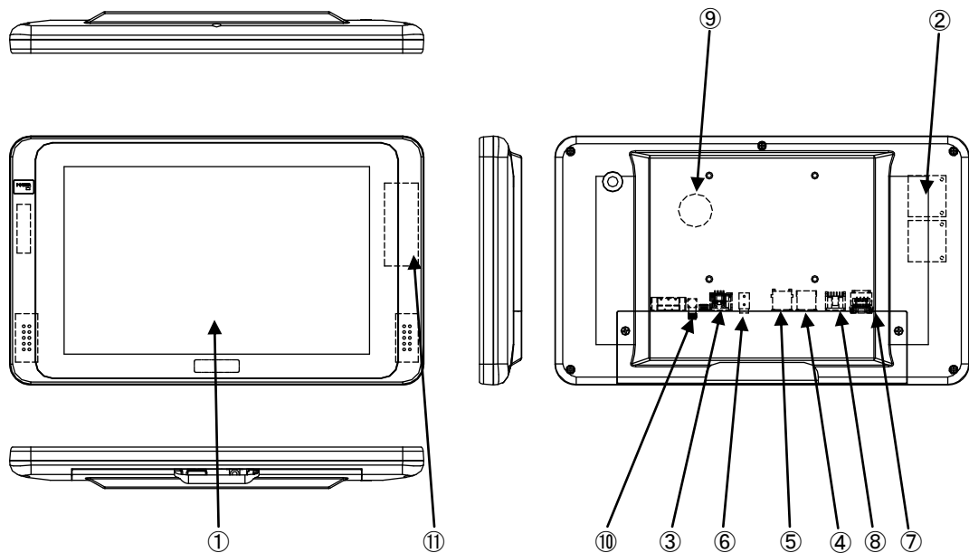
図 4-1. 外形図 (AS4-101BN)
