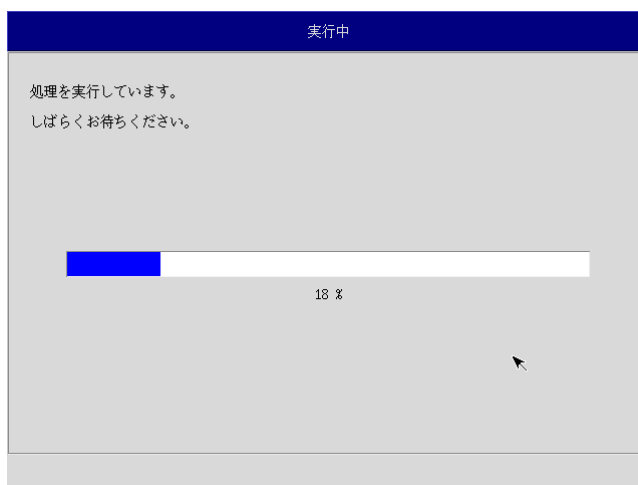
図 5-3-5. 実行中画面
