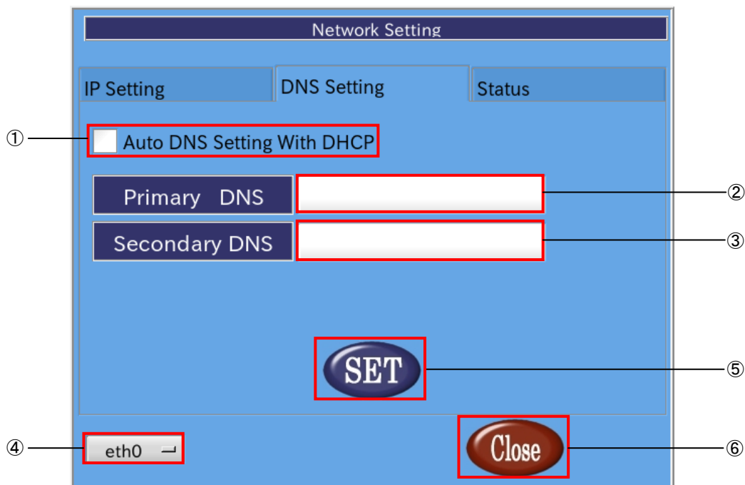
図 2-3-1-2. DNS の設定
