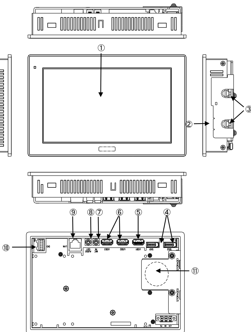
図 3-1-1. 外形図 (APS4-070BN)
