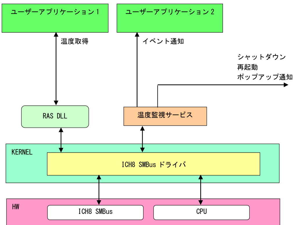
図 4-8-2-1. RAS DLL
