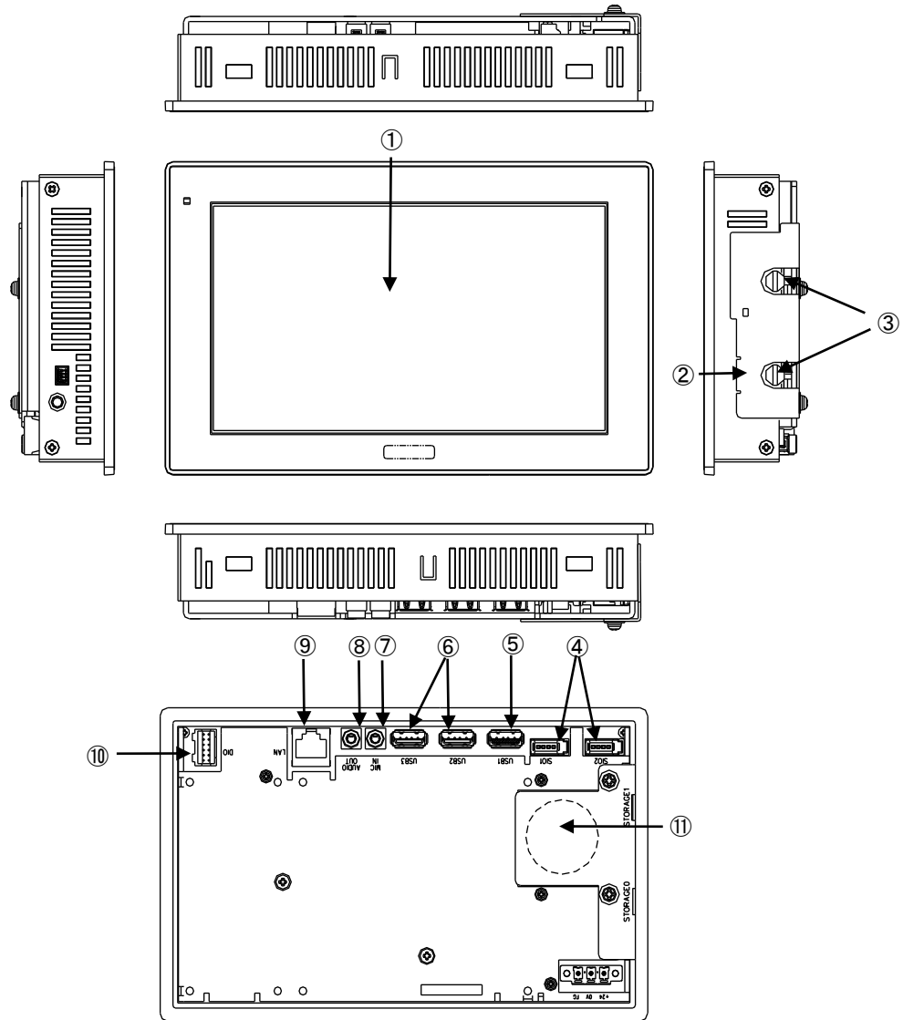
図 4-1. 外形図 (APS4-070Bx)
