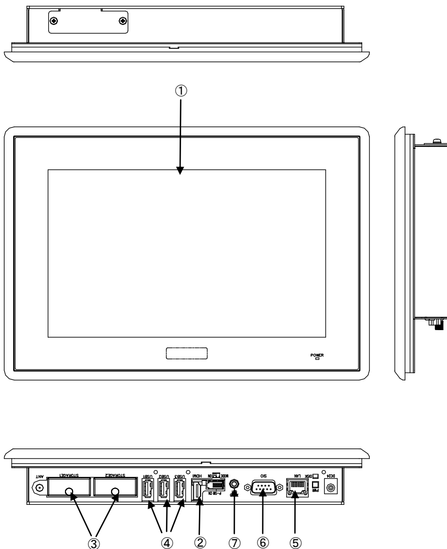
図 3-1-1. 外形図 (APL4-101BN)
