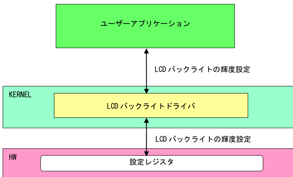
図 5-3-2-1. LCD バックライトドライバ
