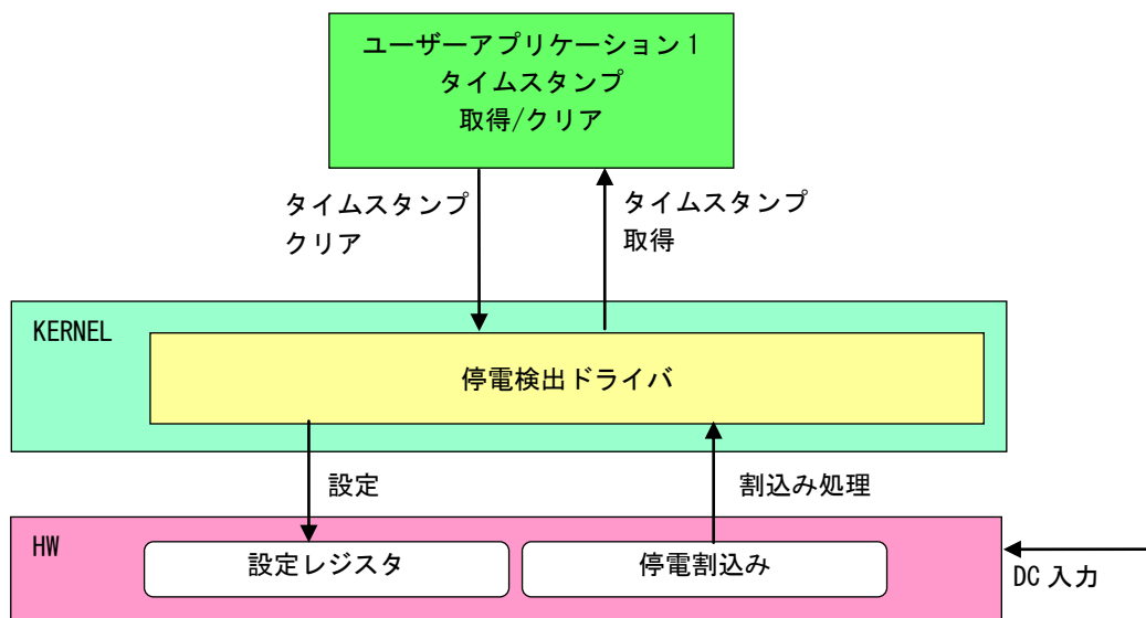
図 5-8-2-1. 停電検出ドライバ
