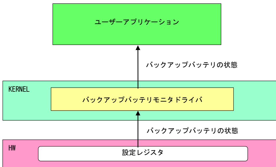
図 5-10-2-1. バックアップバッテリーモニタドライバ
