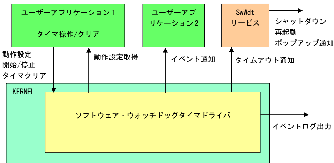
図 5-5-2-1. ソフトウェア・ウォッチドッグタイマドライバ
