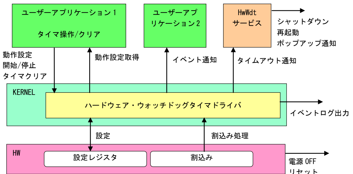
図 5-4-2-1. ハードウェア・ウォッチドッグタイマドライバ
