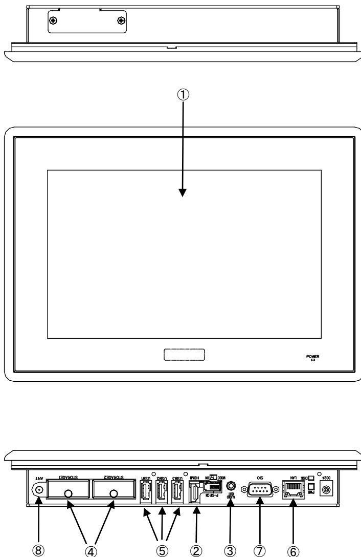
図 4-1. 外形図 (APL4-101BN)
