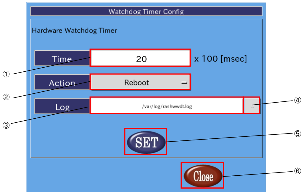
図 2-3-6-1. ハードウェア・ウォッチドッグタイマの設定
