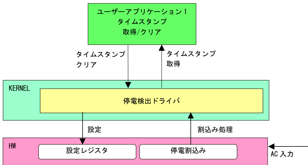
図 5-11-2-1. 停電検出ドライバ
