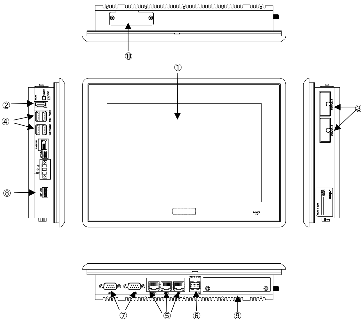
図 3-1-1. 外形図 (AP4-101AN)
