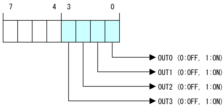
図 5-3-1-2. 出力データ
