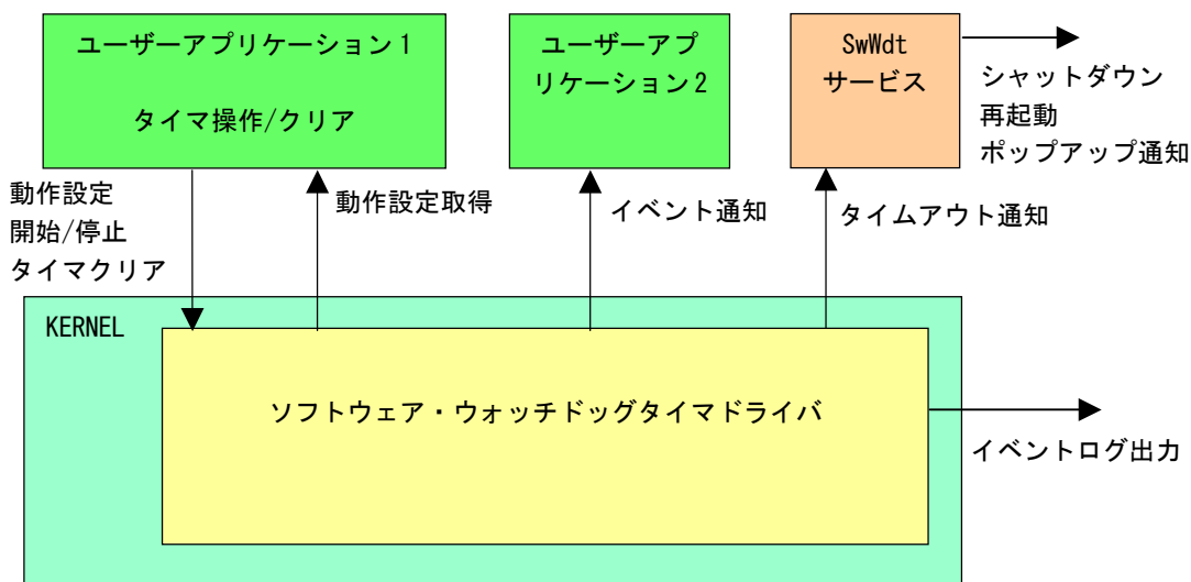
図 5-8-2-1. ソフトウェア・ウォッチドッグタイマドライバ
