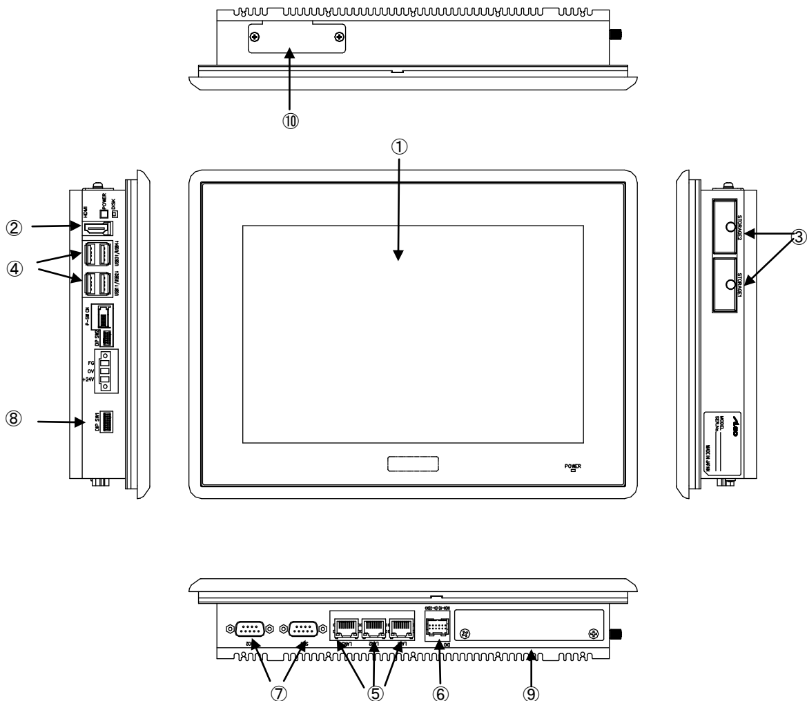
図 4-1. 外形図 (AP4-101AN)
