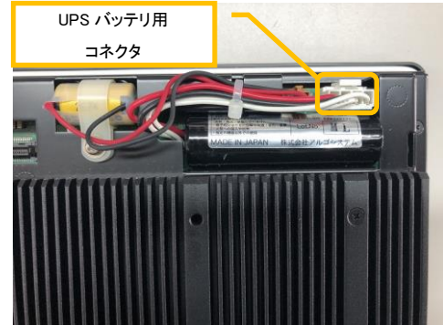
UPS バッテリーを取外す
