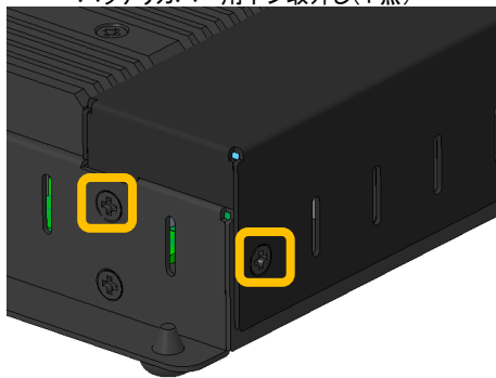
バッテリーカバー用ネジ取外し(4点)
