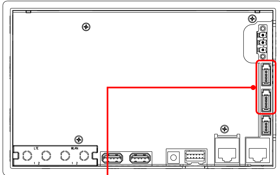
シリアルコネクタ (RS-232C) (上側: SIO1, 下側: SIO2)
