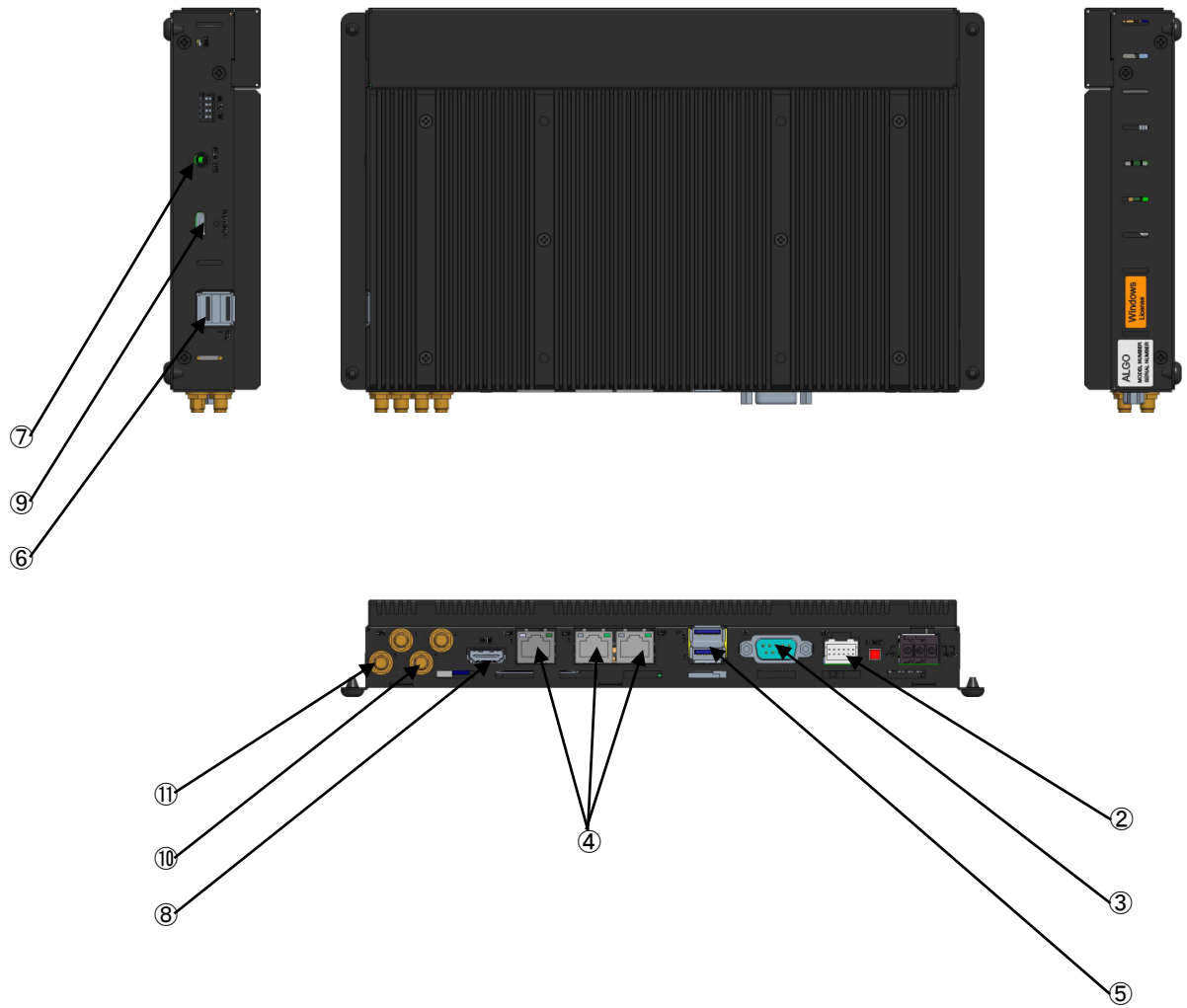
図 3-1-3. 外形図 (EC4C-100AT)
