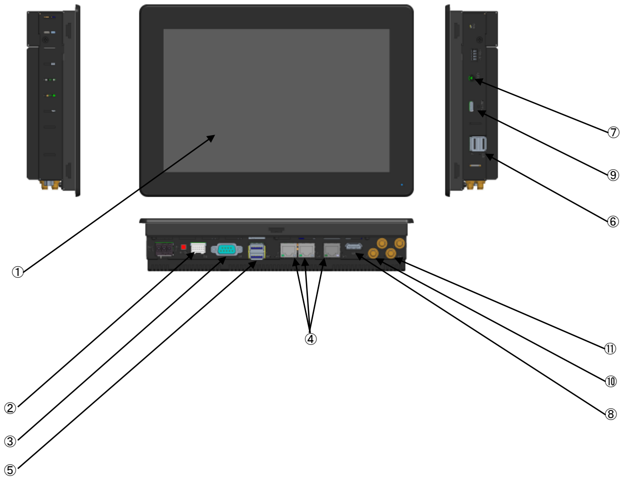
図 3-1-2. 外形図 (NP4C-101A)
