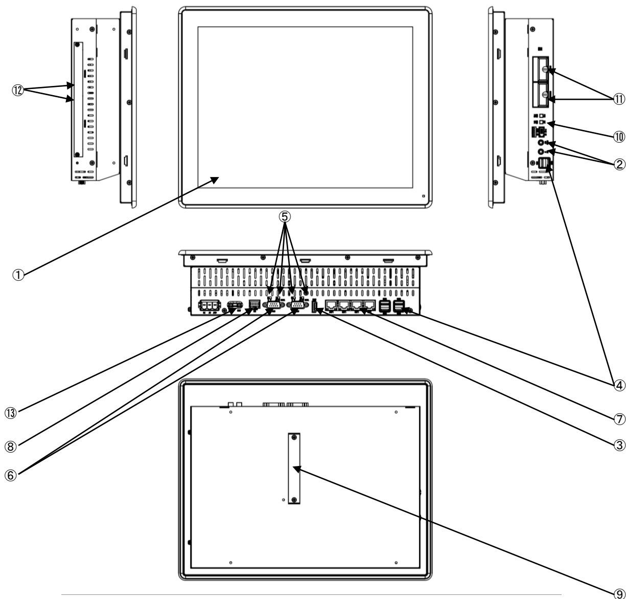
図 3-1-1. 外形図 (NP7A-150AN)
