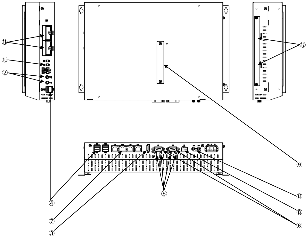
図 3-1-2. 外形図 (EC7A-100A)
