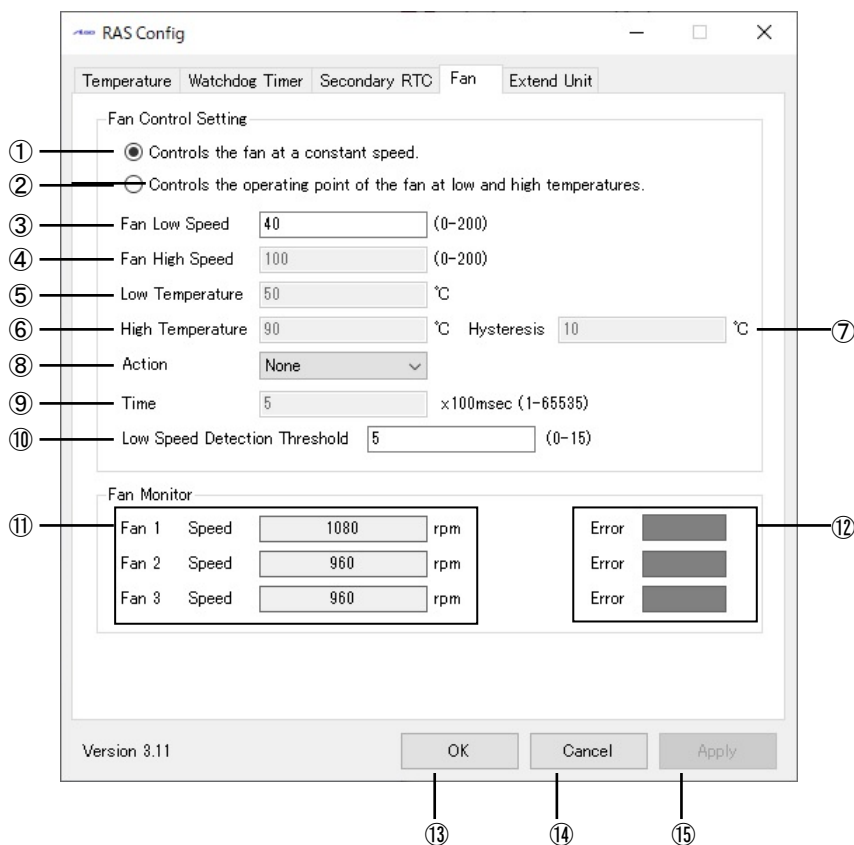
図 2-11-10-1. Fan Control Configuration
