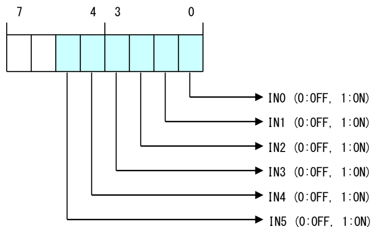
図 4-3-1-1. 入力データ
