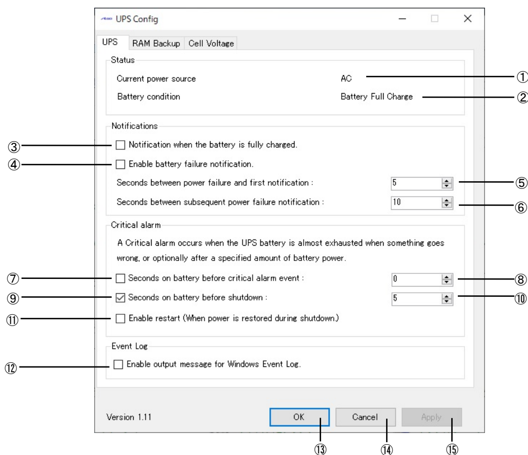
図 2-12-2-1. UPS
