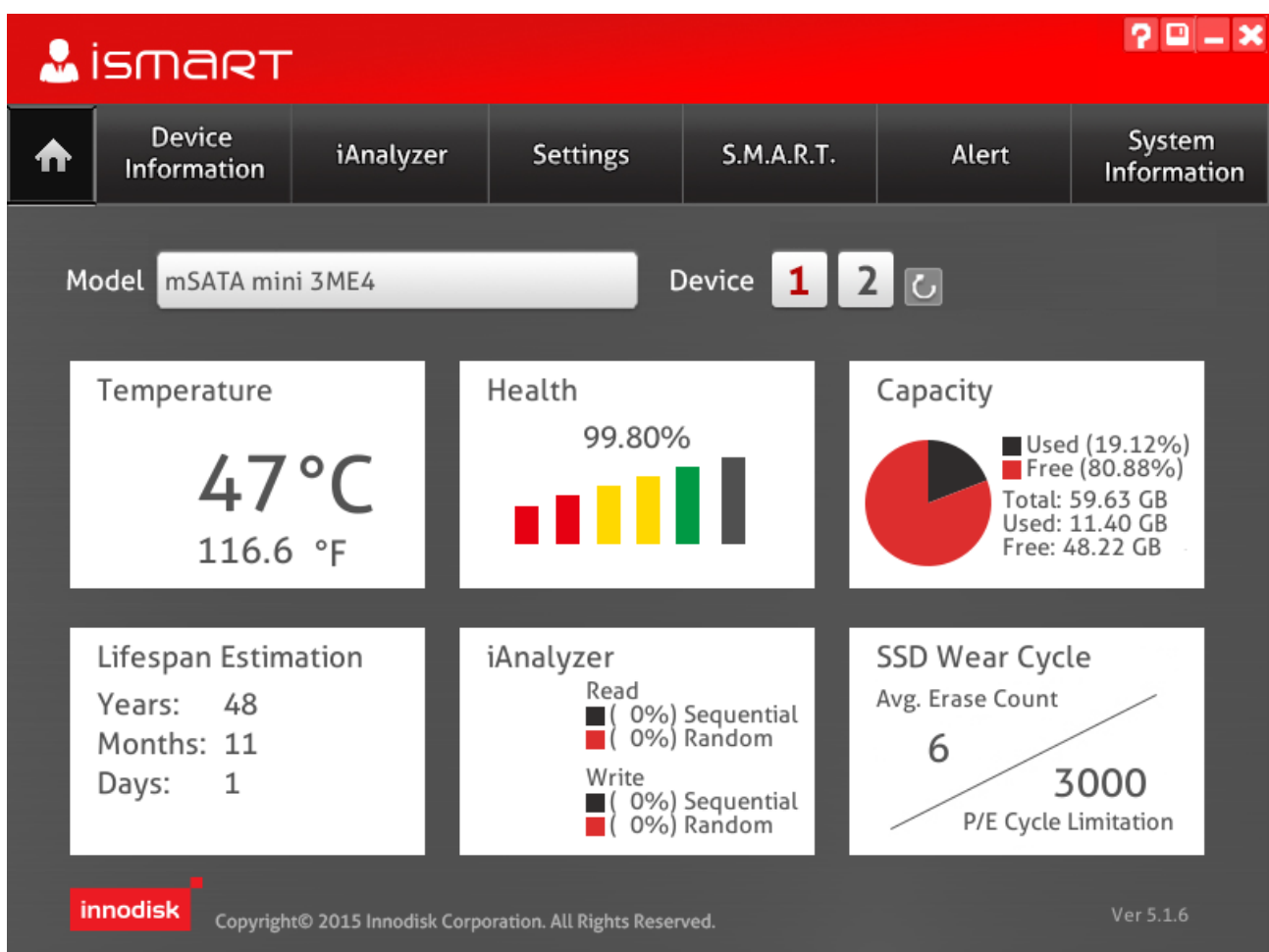
図 2-14-1-1. iSMART 画面
