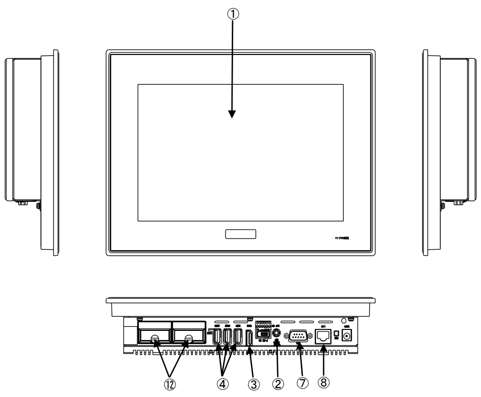
図 3-1-3. 外形図 (APL4A-101BN)
