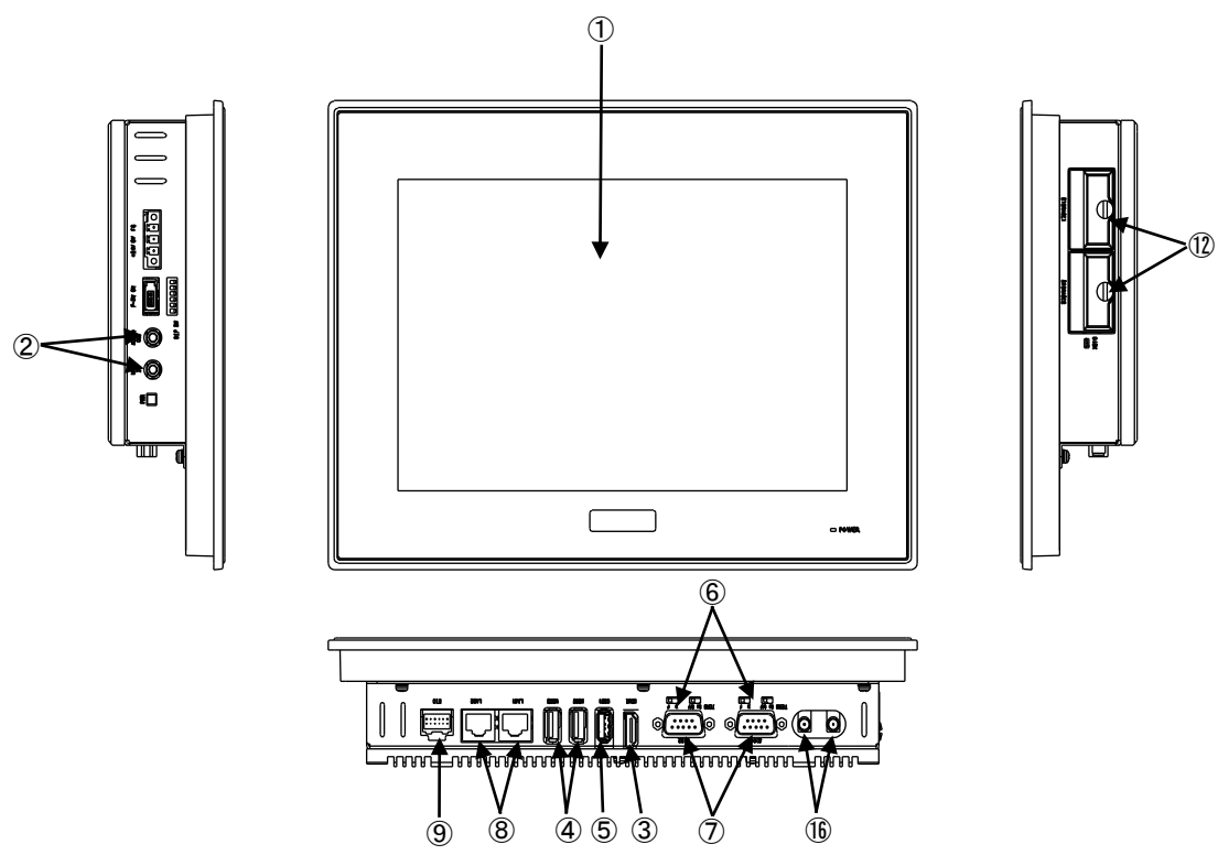
図 3-1-2. 外形図 (APS4A-101BN)
