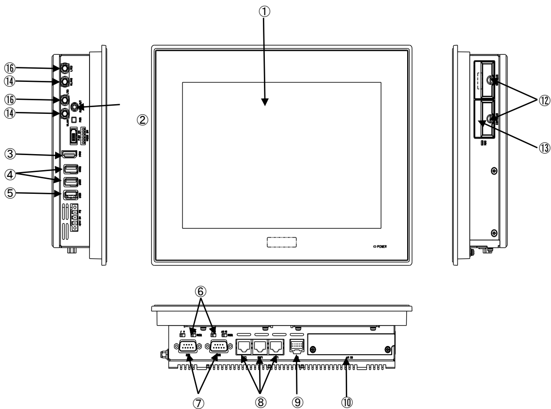
図 3-1-5. 外形図 (AP4A-101CN)
