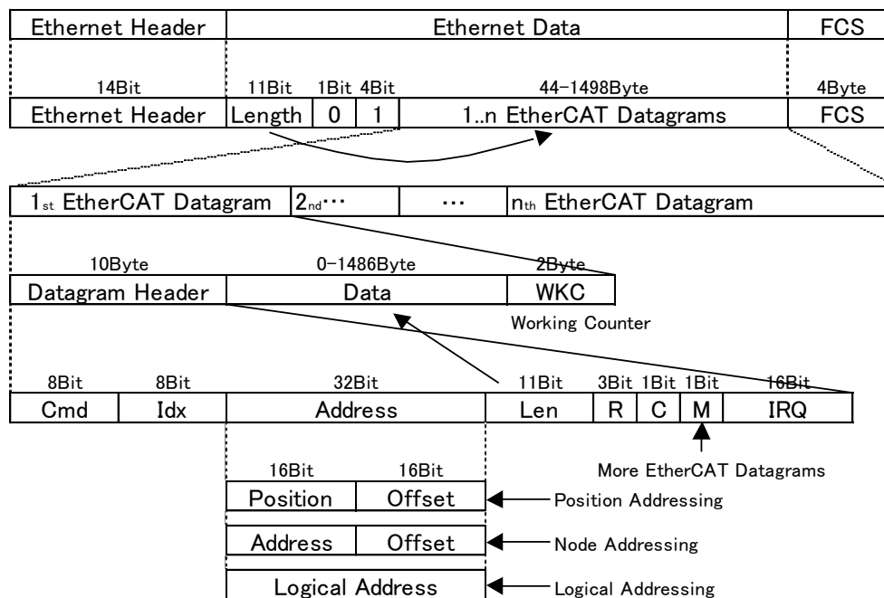
図 3-3-2-2 EtherCAT Datagram
