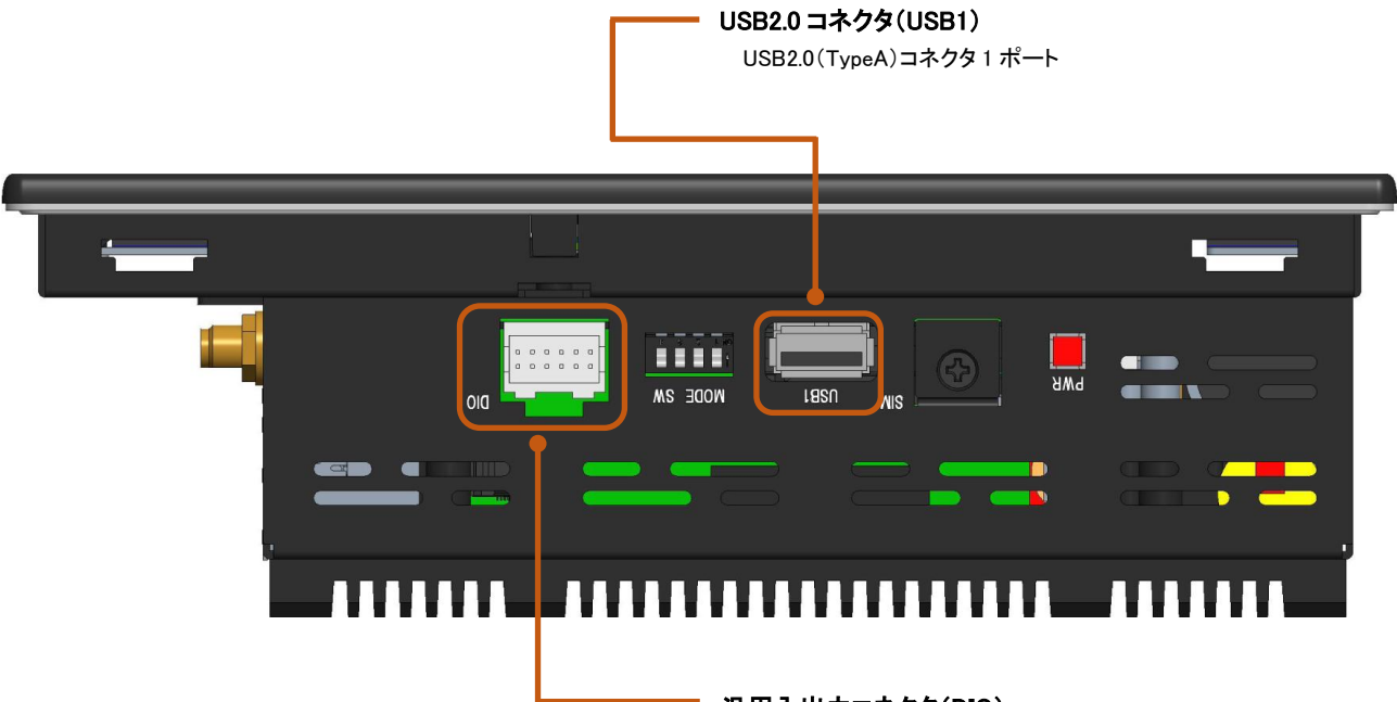
汎用入出力コネクタ(DIO) 接続については「第 4 章 接続」を参照してください
