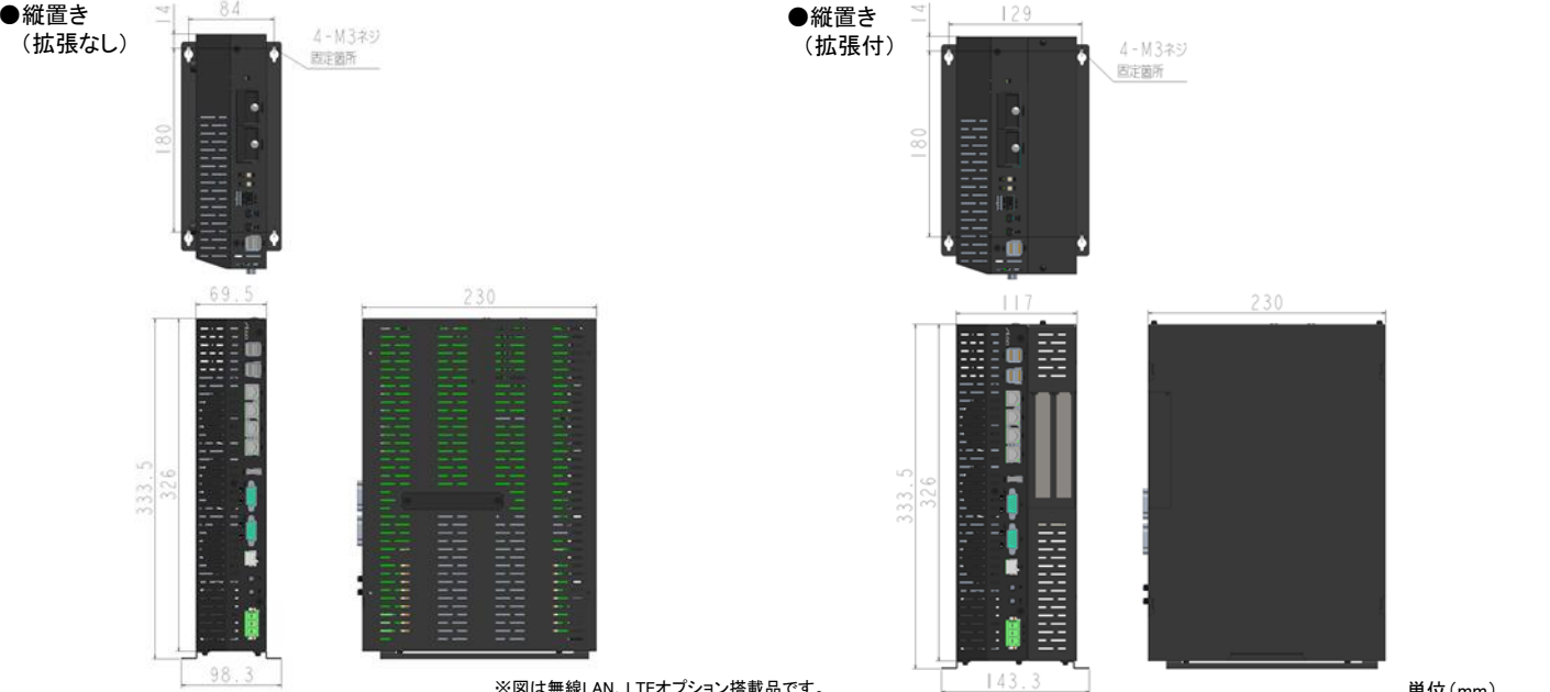
※図は無線LAN、LTEオプション搭載品です。ファン搭載モデルとファン非搭載モデルでは筐体のスロット数が異なります。 単位(mm)
