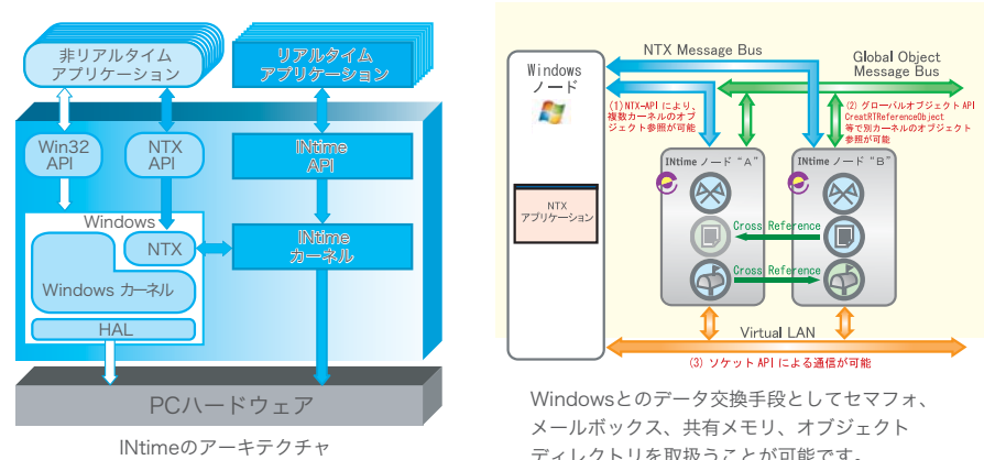
マルチコアCPUとINtimeの動作モード
