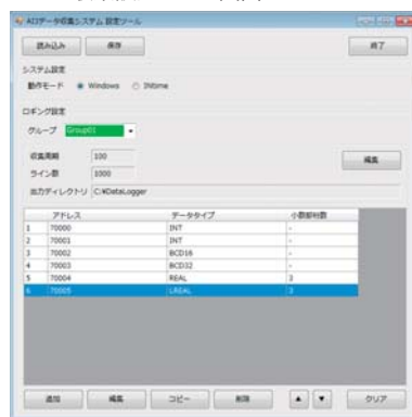
データ収集設定ツール画面
